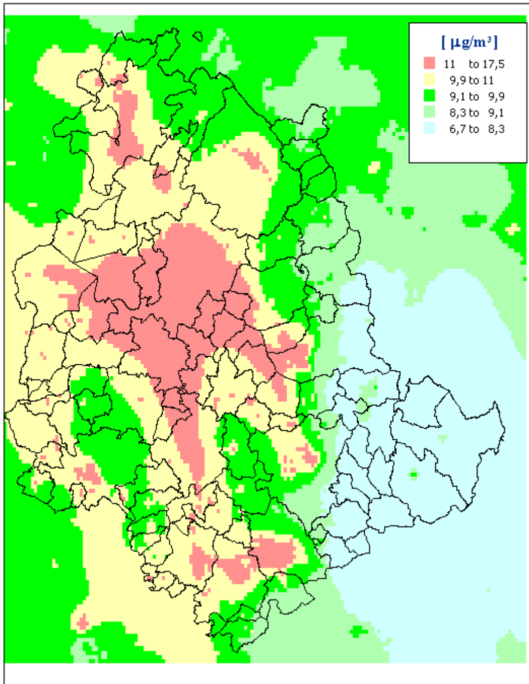
Figura 66 – Media annuale delle concentrazioni di PM 2,5 valutate con il modello Chimere (µg/m 3 ) per l'anno 2025 in Scenario Tendenziale
