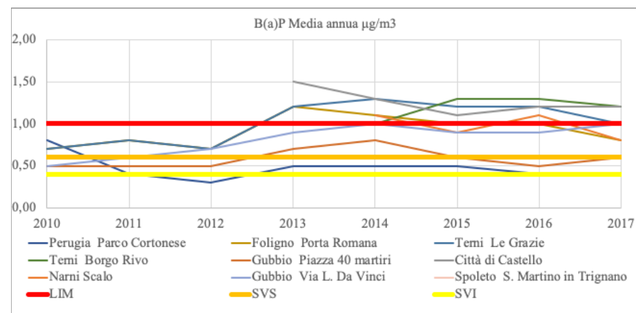
Figura 13 - Rete di rilevamento della qualità dell'aria: media annuale B(a)P
