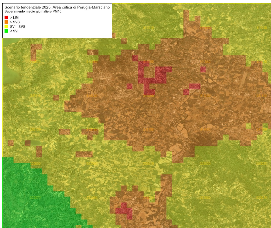
Figura 110 – Superamenti della media giornaliera di PM 10 valutate con il modello Chimere ( \mu\text{g}/\text{m}^3 ) per l'anno 2025 in Scenario Tendenziale per l'area critica Perugia e Marsciano
