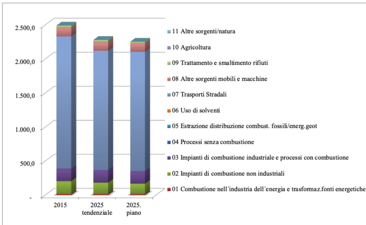
Figura 83 – Andamento delle emissioni totali (Mg) di ossidi di azoto (NO x ) negli scenari tendenziale regionale e di piano per il comune di Perugia
