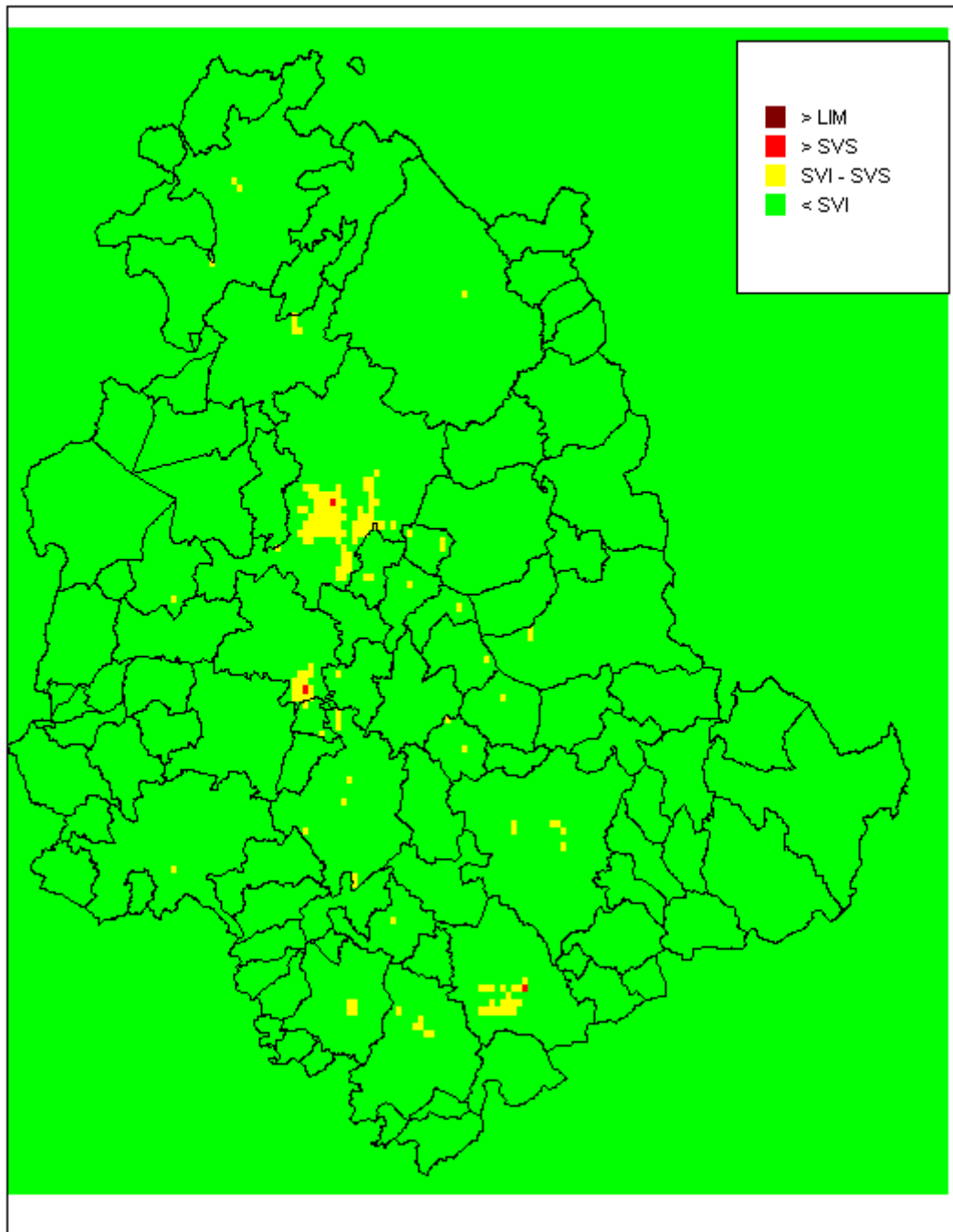
Figura 63 – Media annuale delle concentrazioni di PM 10 totale valutate con il modello Chimere per l'anno 2025 in Scenario Tendenziale con riferimento alle soglie legislative
