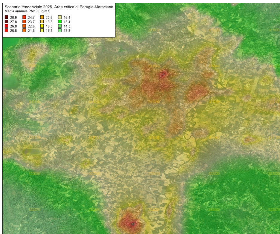
Figura 107 – Media annuale delle concentrazioni di PM 10 totale valutate con il modello Chimere ( \mu\text{g}/\text{m}^3 ) per l'anno 2025 in Scenario Tendenziale l'area critica Perugia e Marsciano
