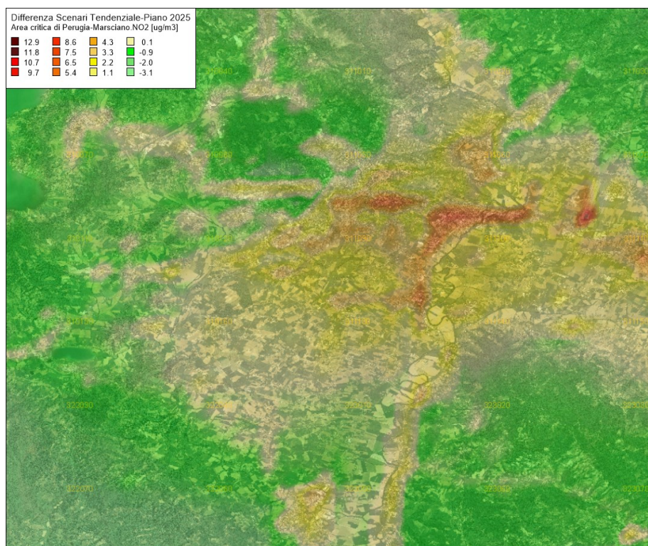
Figura 116 – Riduzione nella media annuale delle concentrazioni di biossido di azoto NO 2 valutate con il modello Chimere (µg/m 3 ) per l'anno 2025 in Scenario di Piano rispetto allo Scenario Tendenziale per l'area critica Perugia e Marsciano
