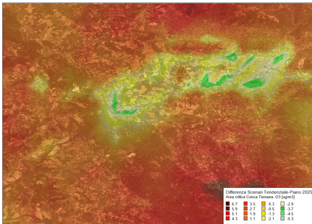
Figura 105 – Variazione nella media annuale delle concentrazioni di ozono ( O_3 ) valutate con il modello Chimere ( \mu g/m^3 ) per l'anno 2025 in Scenario di Piano rispetto allo Scenario Tendenziale per l'area critica conca ternana
