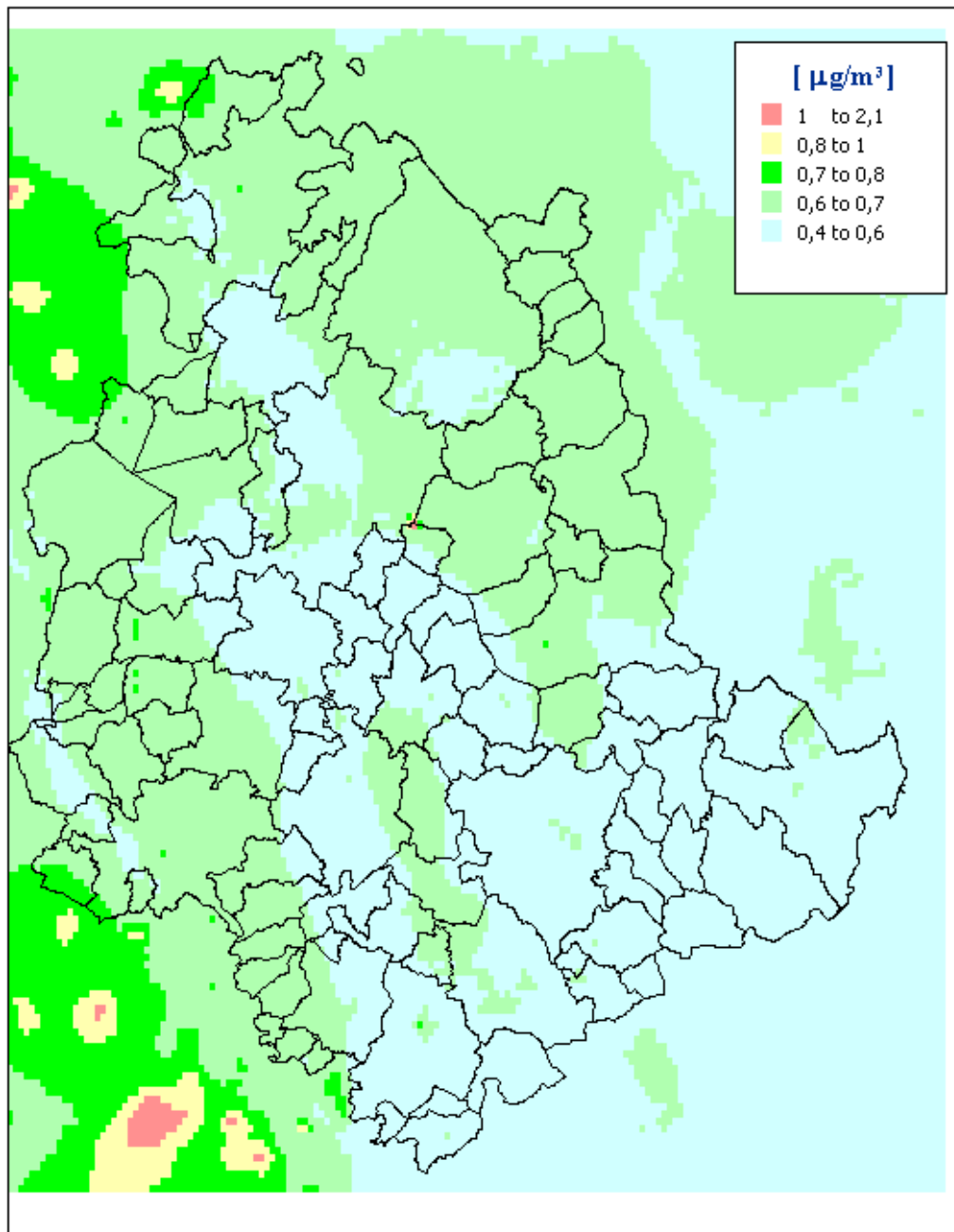
Figura 35 – Media annuale delle concentrazioni di biossido di zolfo (SO 2 ) valutate con il modello Chimere (µg/m 3 ) per l'anno 2015
