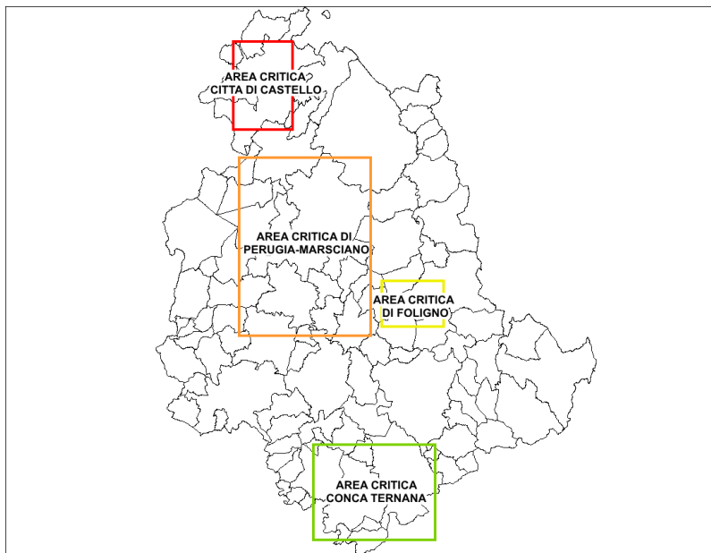
Figura 80 – Aree di applicazione del modello Chimere per l'anno 2025 in Scenario di Piano
