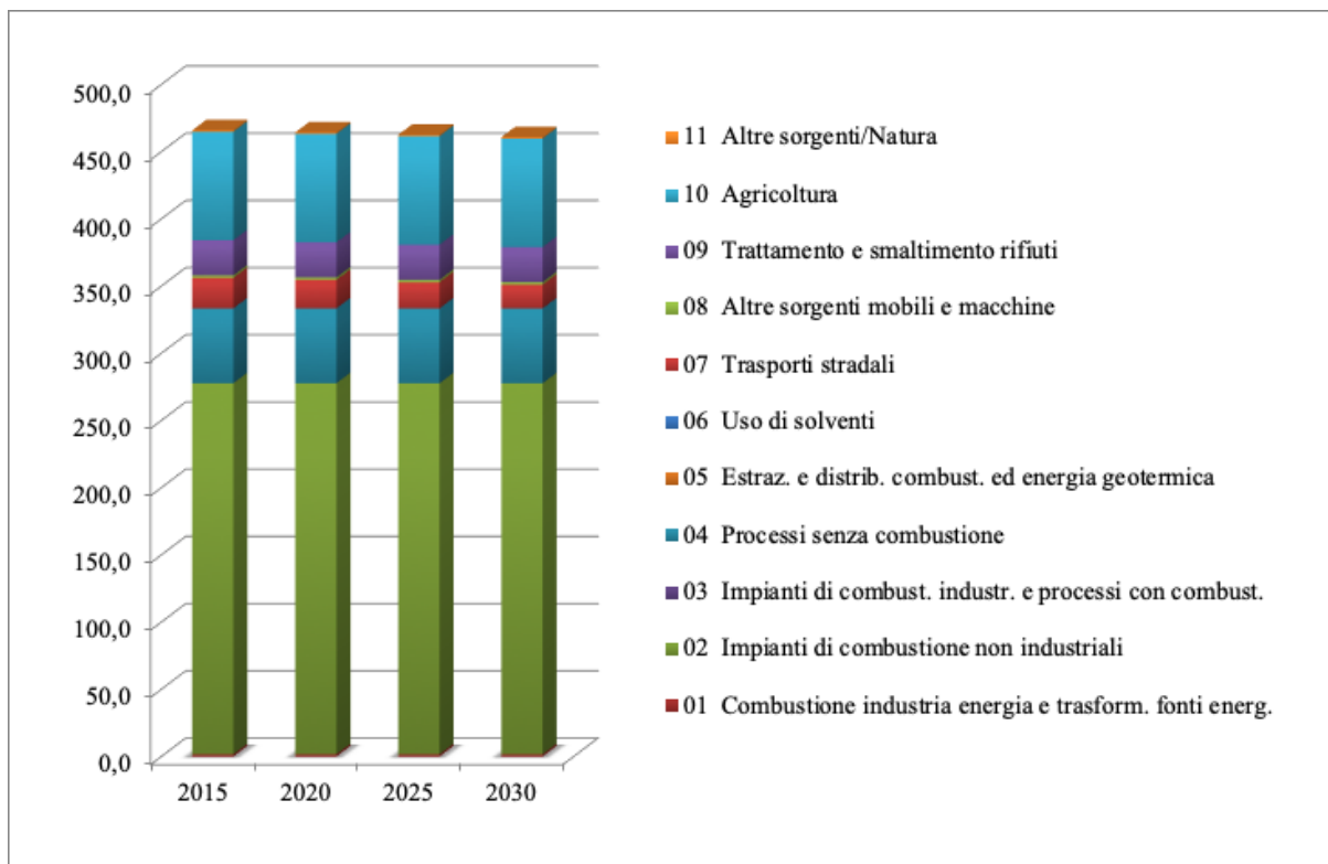
Figura 59 – Andamento delle emissioni totali (Mg) di particelle con diametro inferiore a 10 micron (PM 10 ) nello scenario tendenziale regionale per il comune di Spoleto
