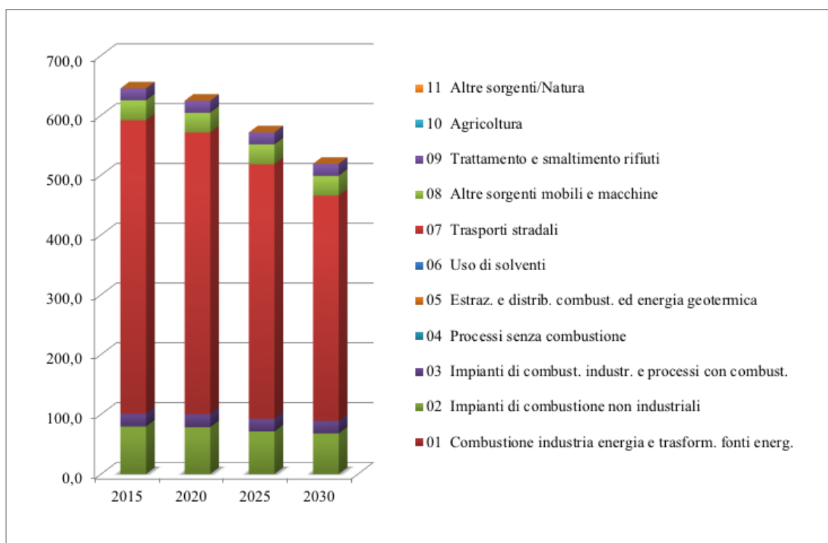
Figura 54 – Andamento delle emissioni totali (Mg) di ossidi di azoto (NO x ) nello scenario tendenziale regionale per il comune di Foligno
