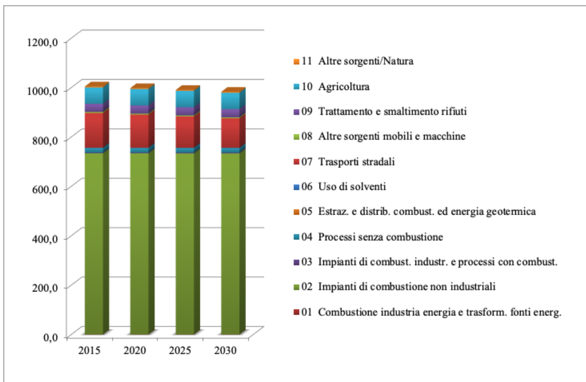
Figura 49 – Andamento delle emissioni totali (Mg) di particelle con diametro inferiore a 10 micron (PM 10 ) nello scenario tendenziale regionale per il comune di Perugia
