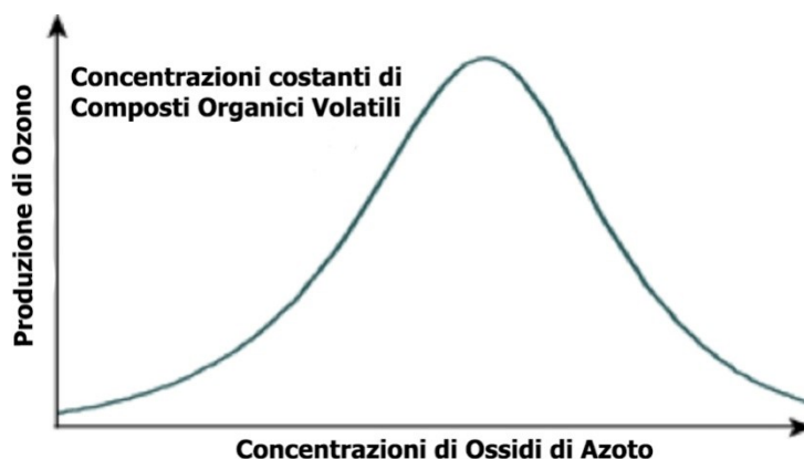
Figura 4 – Efficienza nella formazione di ozono a concentrazione costante di Composti Organici Volatili
