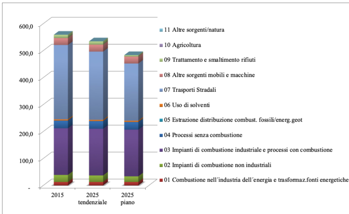
Figura 87 – Andamento delle emissioni totali (Mg) di ossidi di azoto (NO x ) negli scenari tendenziale regionale e di piano per il comune di Narni
