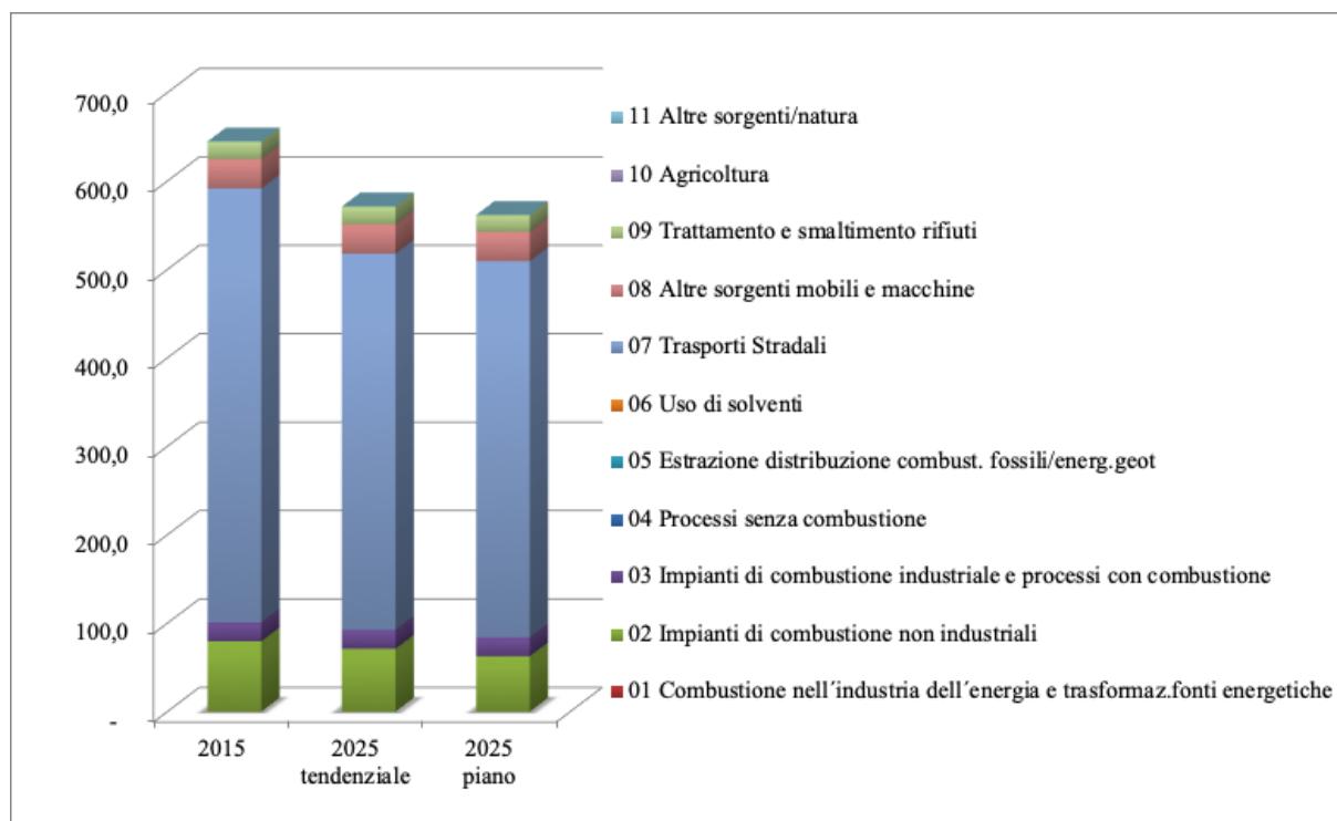
Figura 89 – Andamento delle emissioni totali (Mg) di ossidi di azoto (NO x ) negli scenari tendenziale regionale e di piano per il comune di Foligno
