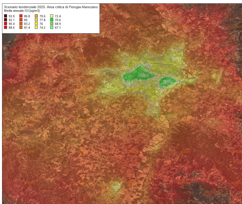
Figura 118 – Media annuale delle concentrazioni di ozono (O 3 ) valutate con il modello Chimere (µg/m³) per l'anno 2025 in Scenario Tendenziale per l'area critica Perugia e Marsciano
