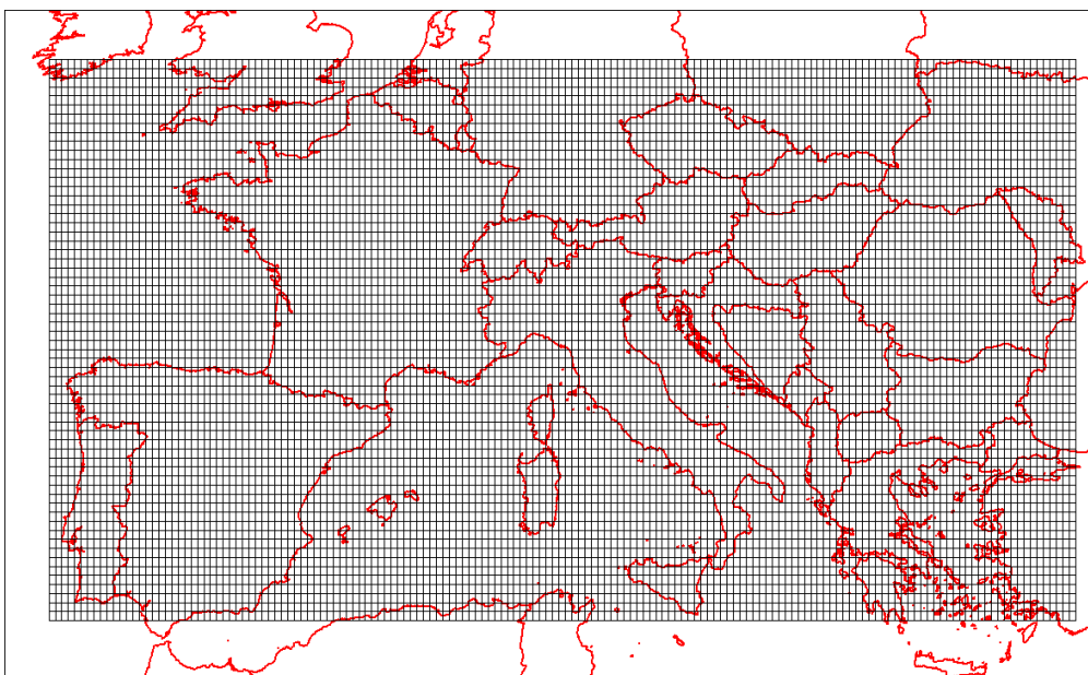
Figura 20 – Dominio geografico scelto per la applicazione di CHIMERE per l'Europa centro-meridionale
