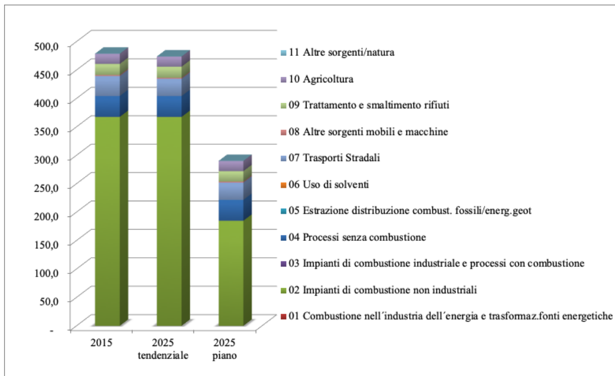
Figura 88 – Andamento delle emissioni totali (Mg) di particelle con diametro inferiore a 10 micron (PM 10 ) negli scenari tendenziale regionale e di piano per il comune di Foligno
