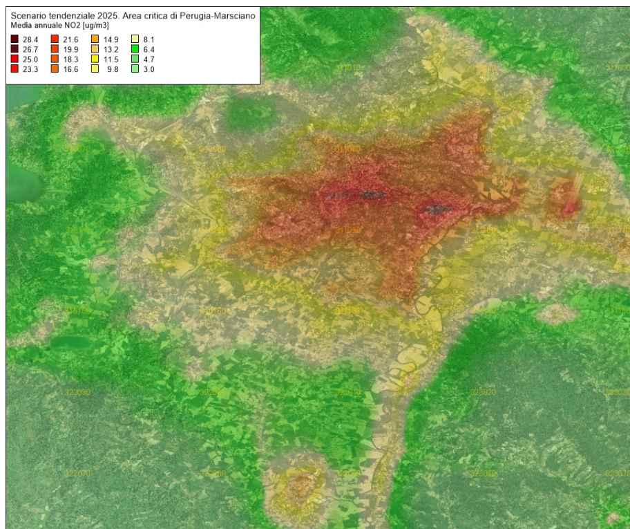
Figura 115 – Media annuale delle concentrazioni di biossido di azoto (NO 2 ) valutate con il modello Chimere (µg/m 3 ) per l'anno 2025 in Scenario Tendenziale l'area critica Perugia e Marsciano
