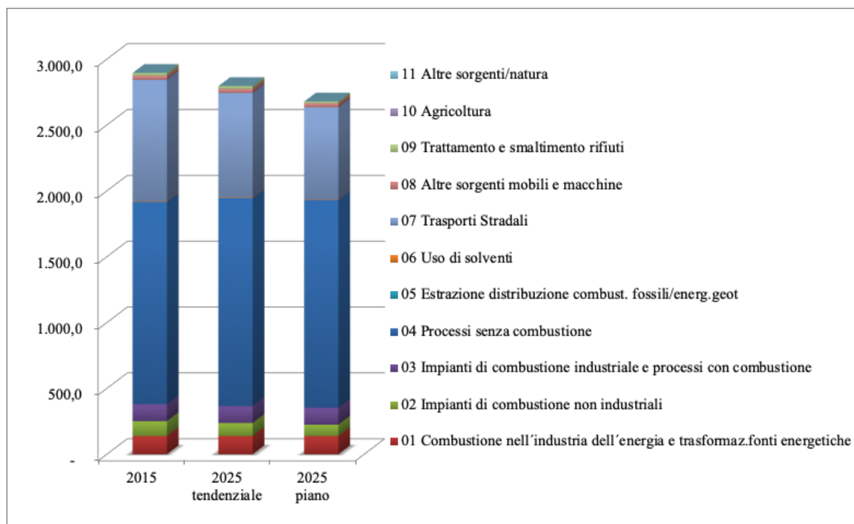
Figura 85 – Andamento delle emissioni totali (Mg) di ossidi di azoto (NO x ) negli scenari tendenziale regionale e di piano per il comune di Terni
