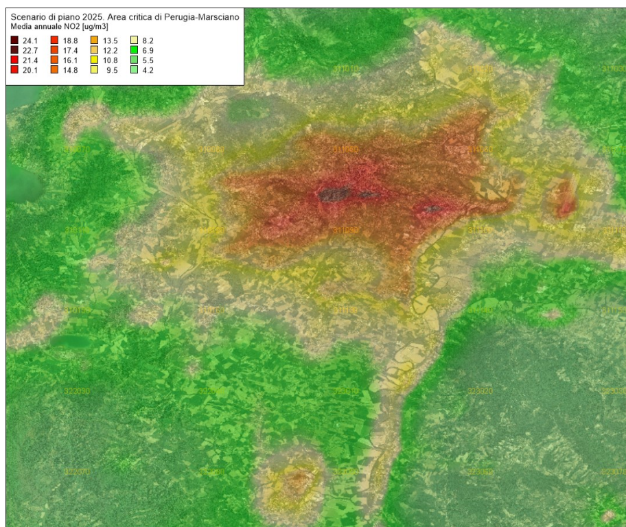
Figura 114 – Media annuale delle concentrazioni di biossido di azoto (NO 2 ) valutate con il modello Chimere (µg/m 3 ) per l'anno 2025 in Scenario di Piano per l'area critica Perugia e Marsciano
