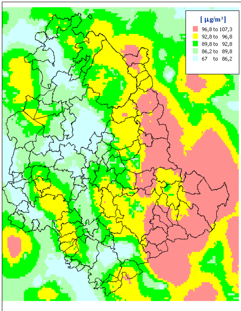
Figura 34 – Media annuale delle concentrazioni di ozono valutate con il modello Chimere (µg/m³) per l'anno 2015
