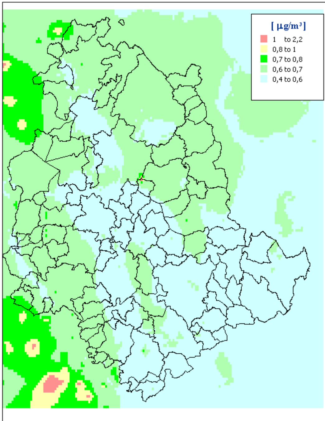
Figura 69 – Media annuale delle concentrazioni di biossido di zolfo (SO 2 ) valutate con il modello Chimere (µg/m 3 ) per l'anno 2025 in Scenario Tendenziale
