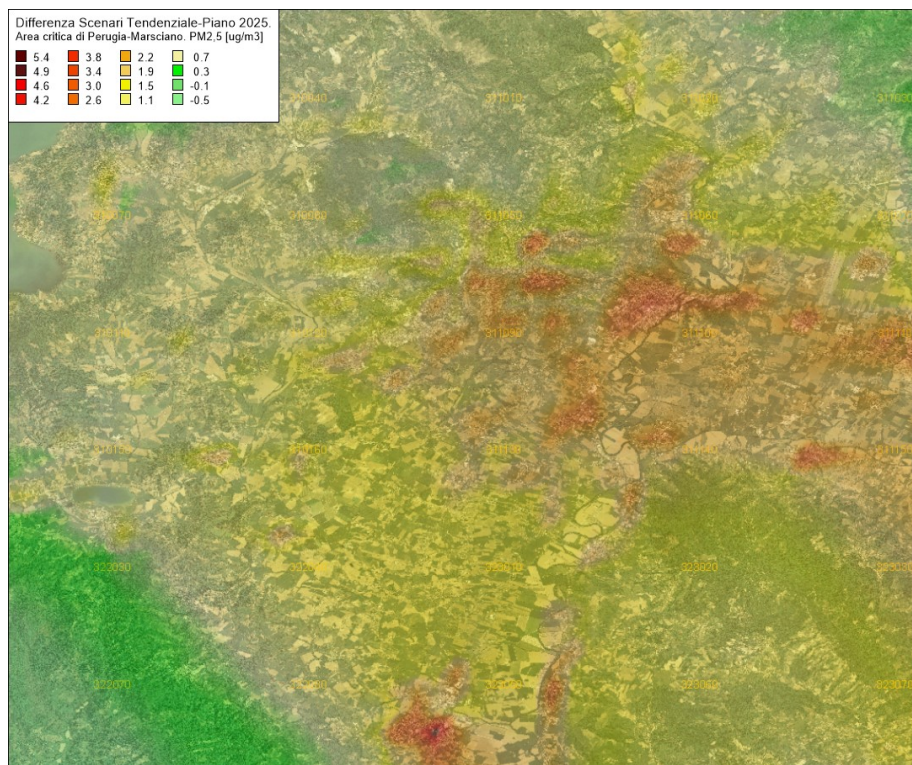
Figura 113 – Riduzione nella media annuale delle concentrazioni di PM 2,5 totale valutate con il modello Chimere (µg/m 3 ) per l'anno 2025 in Scenario di Piano rispetto allo Scenario Tendenziale per l'area critica Perugia e Marsciano
