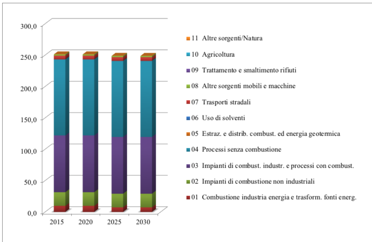
Figura 47 – Andamento delle emissioni totali (kg) di nickel nello scenario tendenziale regionale
