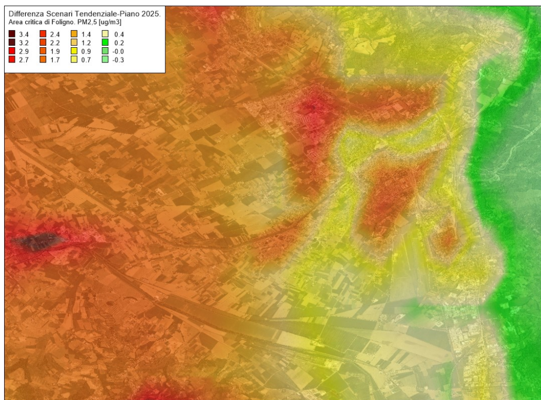
Figura 127 – Riduzione nella media annuale delle concentrazioni di PM 2,5 valutate con il modello Chimere (µg/m³) per l'anno 2025 in Scenario di Piano rispetto allo Scenario Tendenziale per l'area critica Foligno
