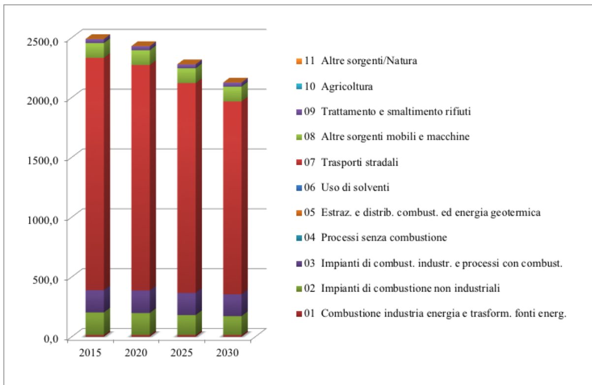
Figura 48 – Andamento delle emissioni totali (Mg) di ossidi di azoto (NO x ) nello scenario tendenziale regionale per il comune di Perugia
