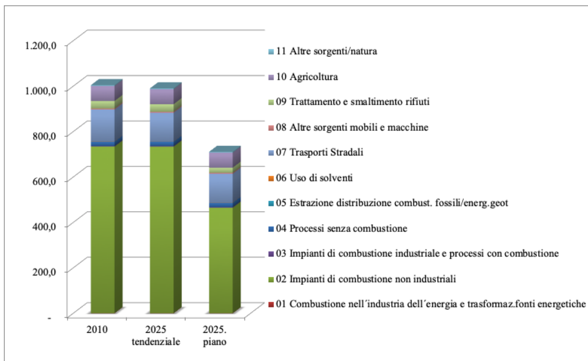
Figura 82 – Andamento delle emissioni totali (Mg) di particelle con diametro inferiore a 10 micron (PM 10 ) negli scenari tendenziale regionale e di piano per il comune di Perugia
