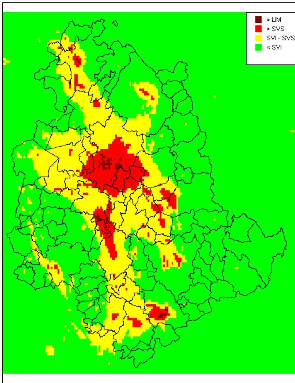
Figura 37 – Stima dei superamenti di soglie di valutazione e valore limite per la media giornaliera del PM 10 valutati con il modello Chimere per l'anno 2015
