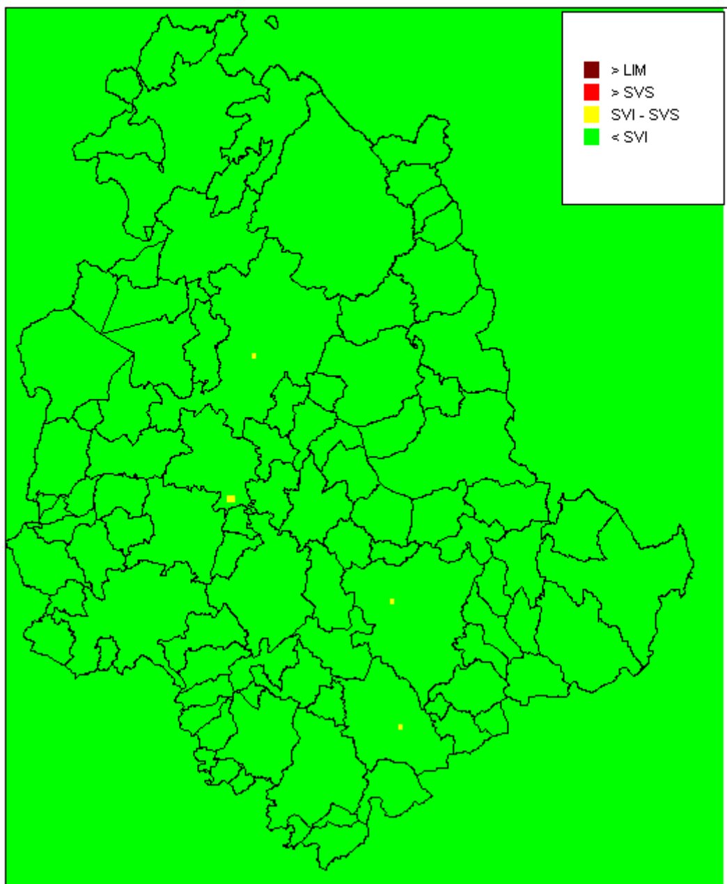
Figura 65 – Media annuale delle concentrazioni di PM 10 antropico valutate con il modello Chimere per l'anno 2025 in Scenario Tendenziale con riferimento alle soglie legislative
