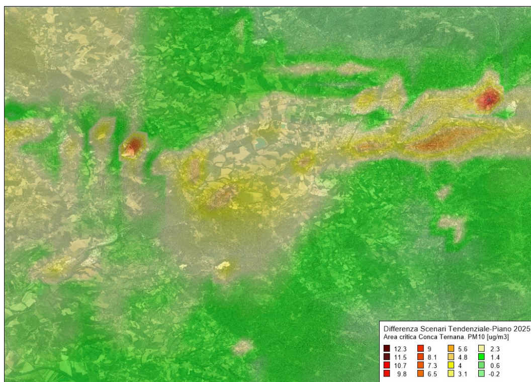
Figura 94 – Riduzione nella media annuale delle concentrazioni di \text{PM}_{10} totale valutate con il modello Chimere ( \mu\text{g}/\text{m}^3 ) per l'anno 2025 in Scenario Tendenziale per l'area critica conca ternana
