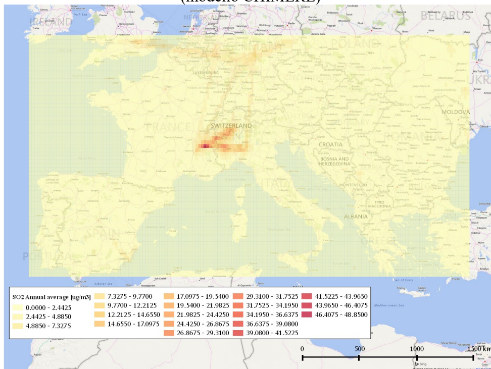
Figura 24 - Media annuale di SO 2 nel 2015 per l'Europa centro-meridionale (modello CHIMERE)
