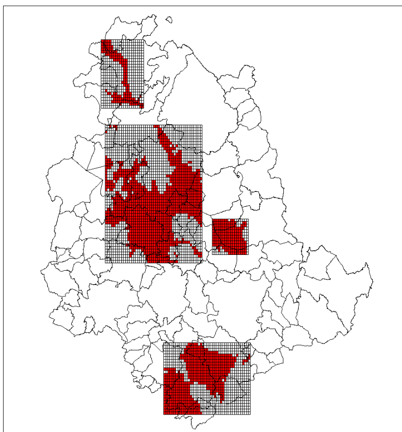
Figura 81 – Maglie di territorio posto a una quota inferiore ai 300 m nelle Aree critiche
