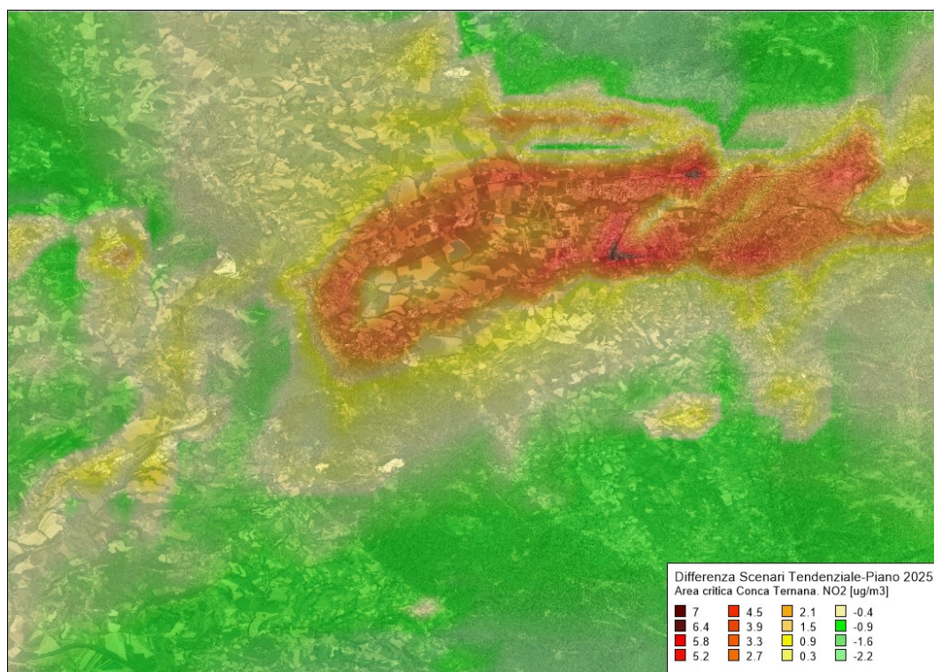
Figura 102 – Riduzione nella media annuale delle concentrazioni di biossido di azoto NO 2 valutate con il modello Chimere (µg/m 3 ) per l'anno 2025 in Scenario di Piano rispetto allo Scenario Tendenziale per l'area critica conca ternana
