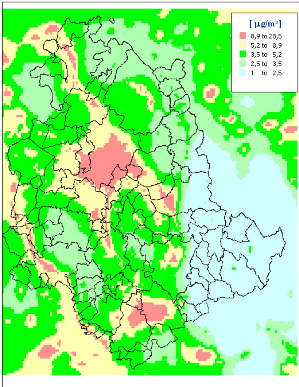
Figura 60 – Media annuale delle concentrazioni di biossido di azoto (NO 2 ) valutate con il modello Chimere (µg/m 3 ) per l'anno 2025 in Scenario Tendenziale
