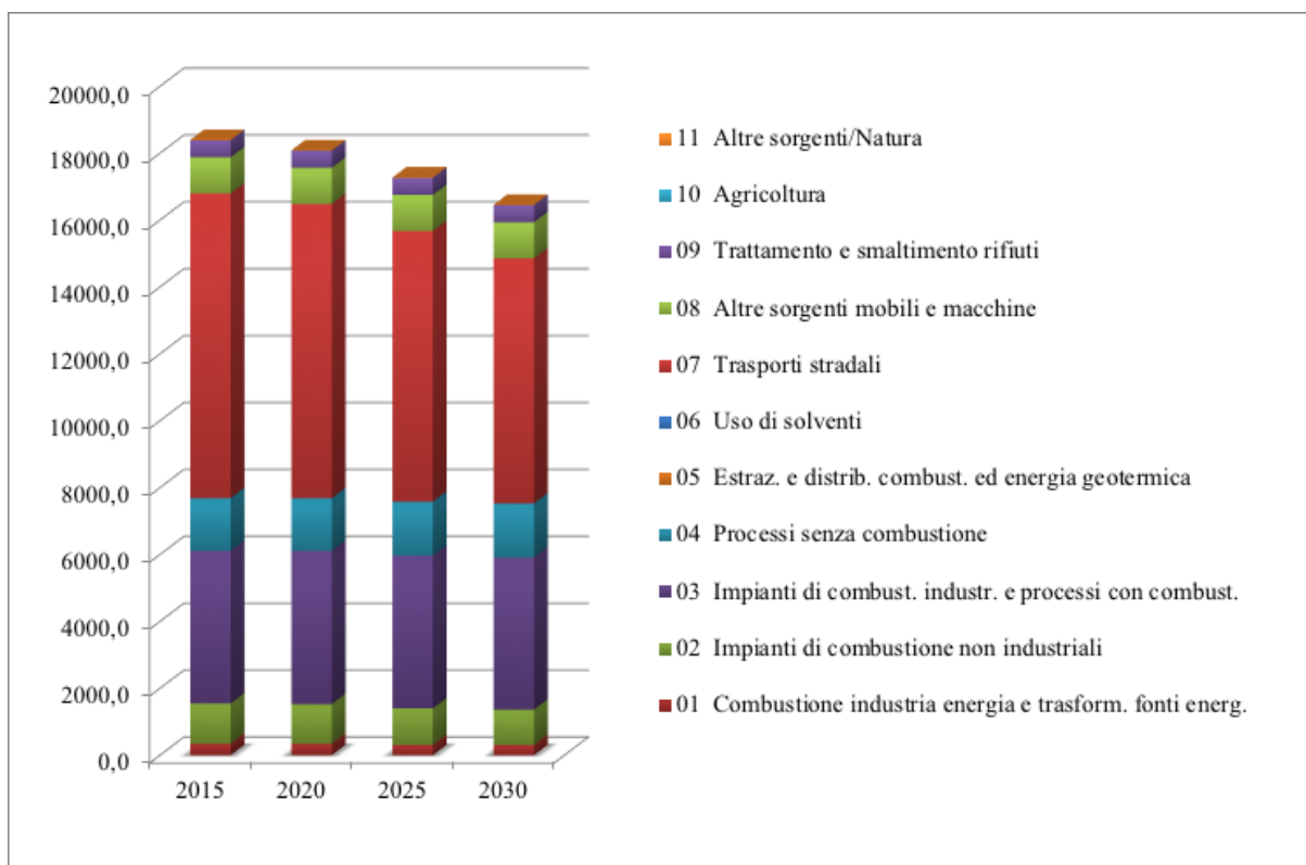
Figura 42 – Andamento delle emissioni totali (Mg) di ossidi di azoto (NO x ) nello scenario tendenziale regionale
