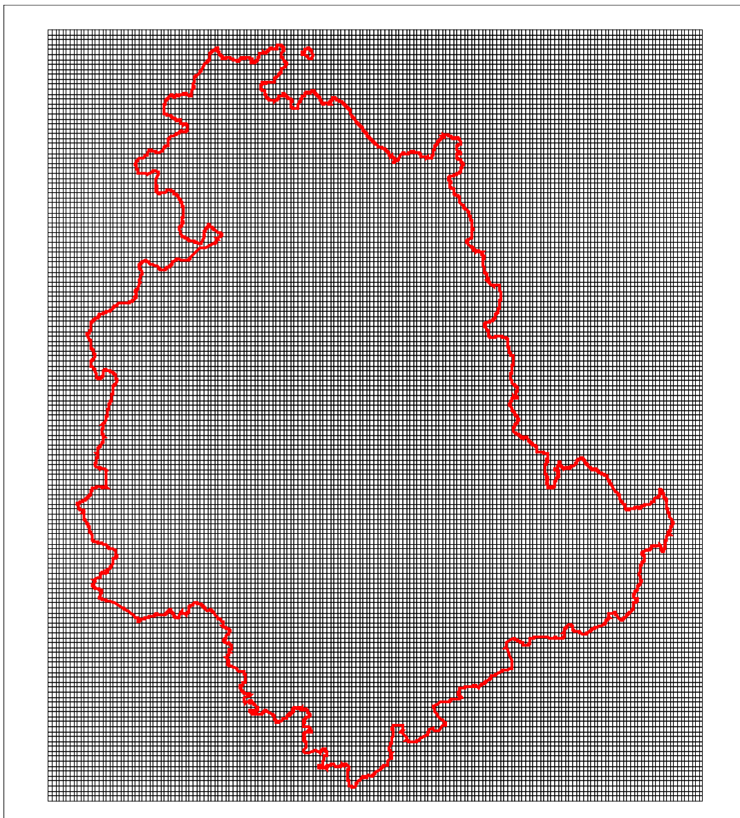
Figura 19 – Griglia utilizzata per la disaggregazione delle emissioni al fine del loro utilizzo nel modello Chimere su tutto il territorio regionale
