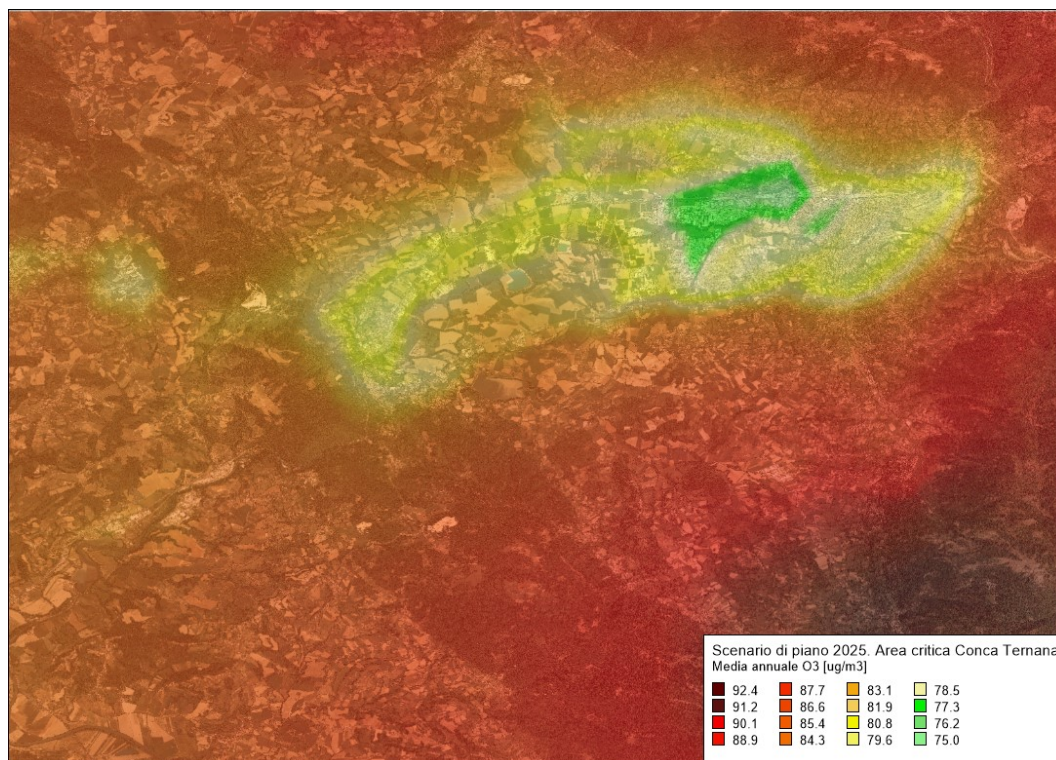
Figura 103 – Media annuale delle concentrazioni di ozono (O 3 ) valutate con il modello Chimere (µg/m 3 ) per l'anno 2025 in Scenario di Piano per l'area critica conca ternana
