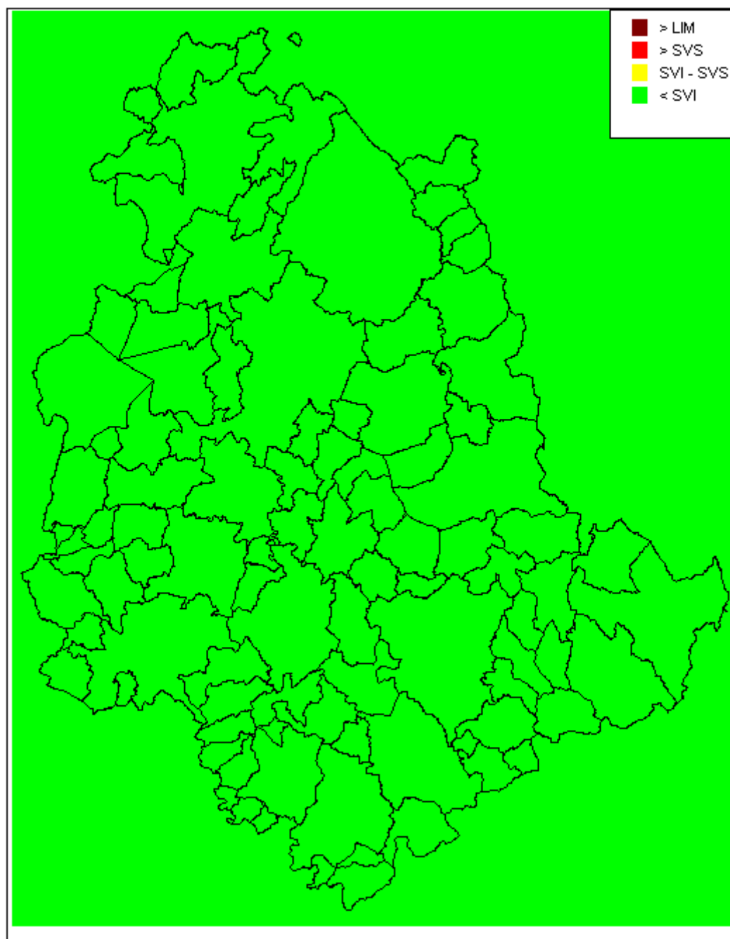
Figura 74 – Stima dei superamenti di soglie di valutazione e valore limite per la media giornaliera degli ossidi di zolfo valutati con il modello Chimere per l'anno 2025 in Scenario Tendenziale
