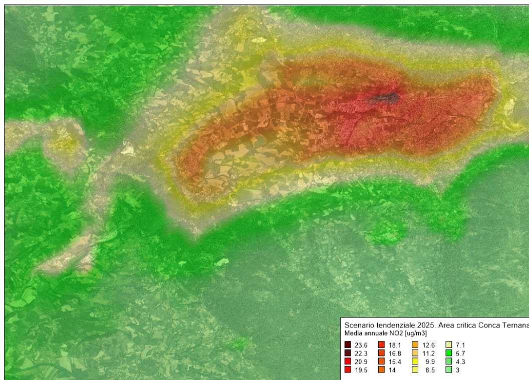
Figura 101 – Media annuale delle concentrazioni di biossido di azoto (NO 2 ) valutate con il modello Chimere (µg/m 3 ) per l'anno 2025 in Scenario Tendenziale per l'area critica conca ternana
