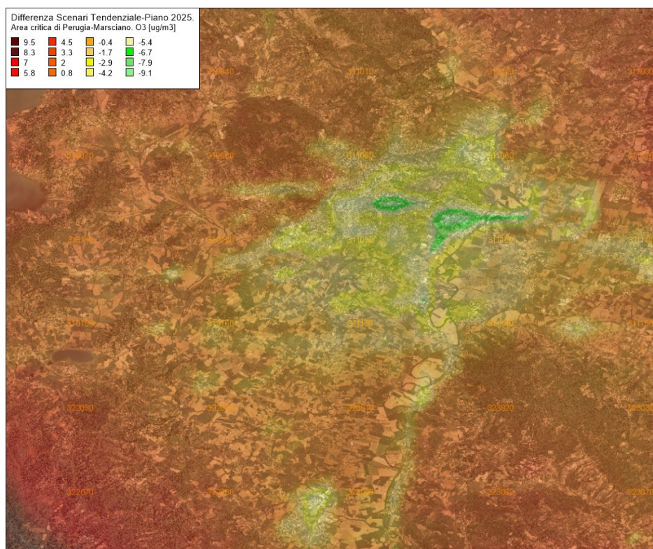
Figura 119 – Variazione nella media annuale delle concentrazioni di ozono ( O_3 ) valutate con il modello Chimere ( \mu g/m^3 ) per l'anno 2025 in Scenario di Piano rispetto allo Scenario Tendenziale per l'area critica Perugia e Marsciano
