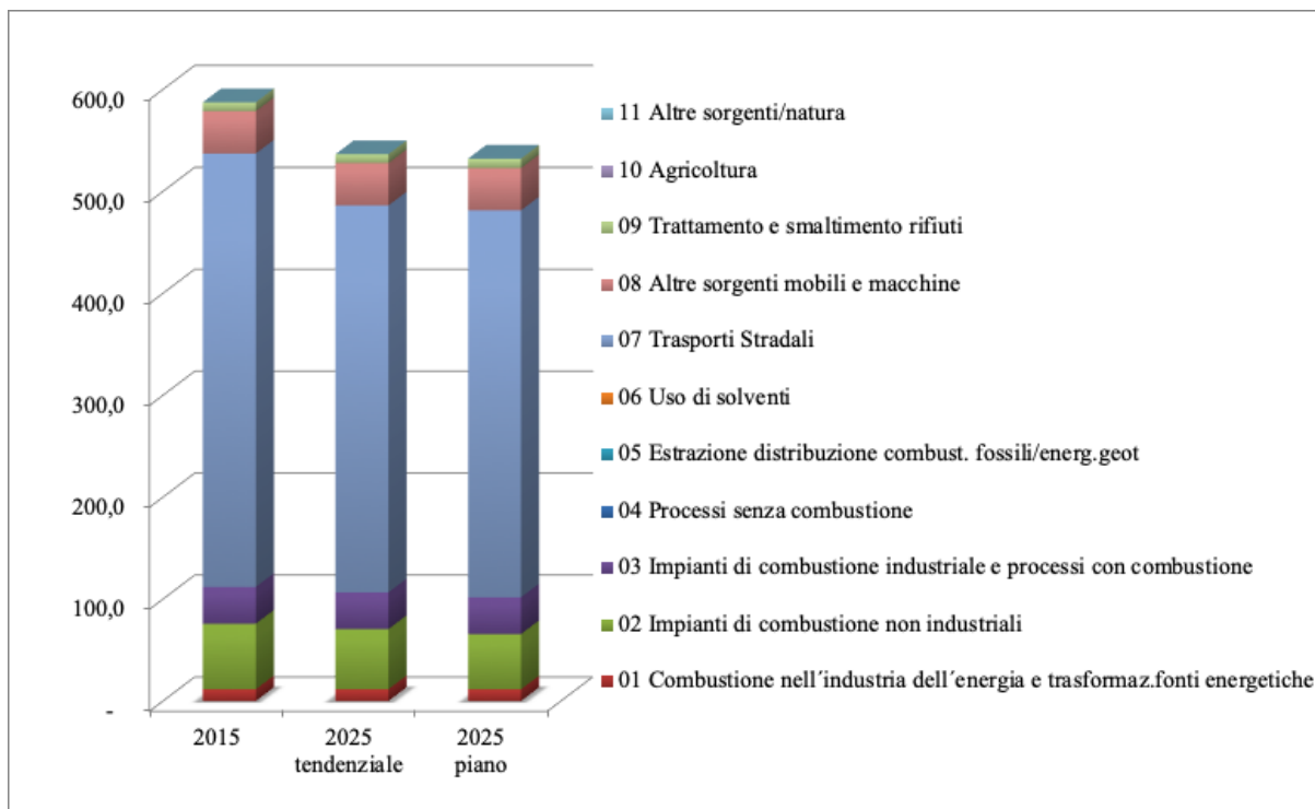
Figura 91 – Andamento delle emissioni totali (Mg) di ossidi di azoto (NO x ) negli scenari tendenziale regionale e di piano per il comune di Città di Castello
