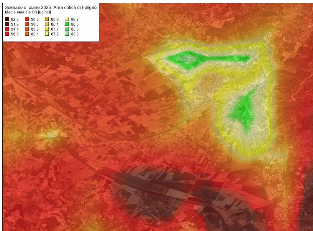
Figura 131 – Media annuale delle concentrazioni di ozono (O 3 ) valutate con il modello Chimere (µg/m 3 ) per l'anno 2025 in Scenario di Piano per l'area critica Foligno
