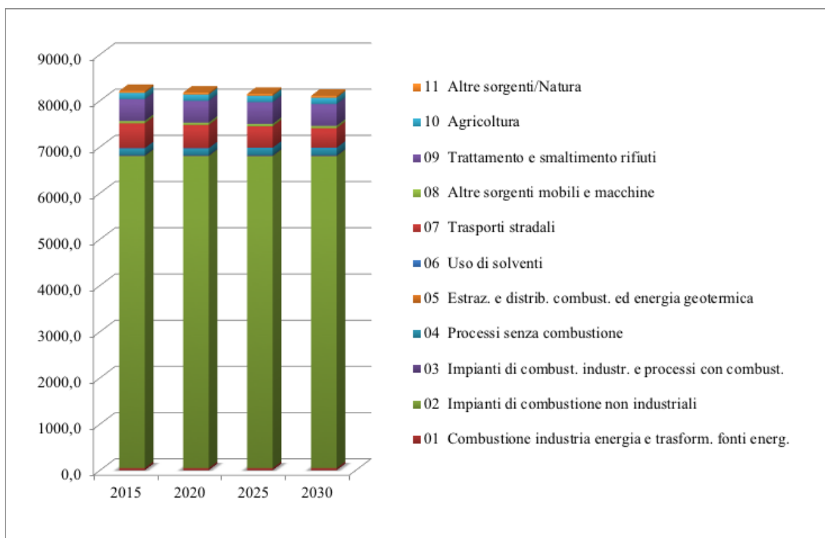
Figura 44 – Andamento delle emissioni totali (Mg) di particelle con diametro inferiore a 2,5 micron (PM 2.5 ) nello scenario tendenziale regionale
