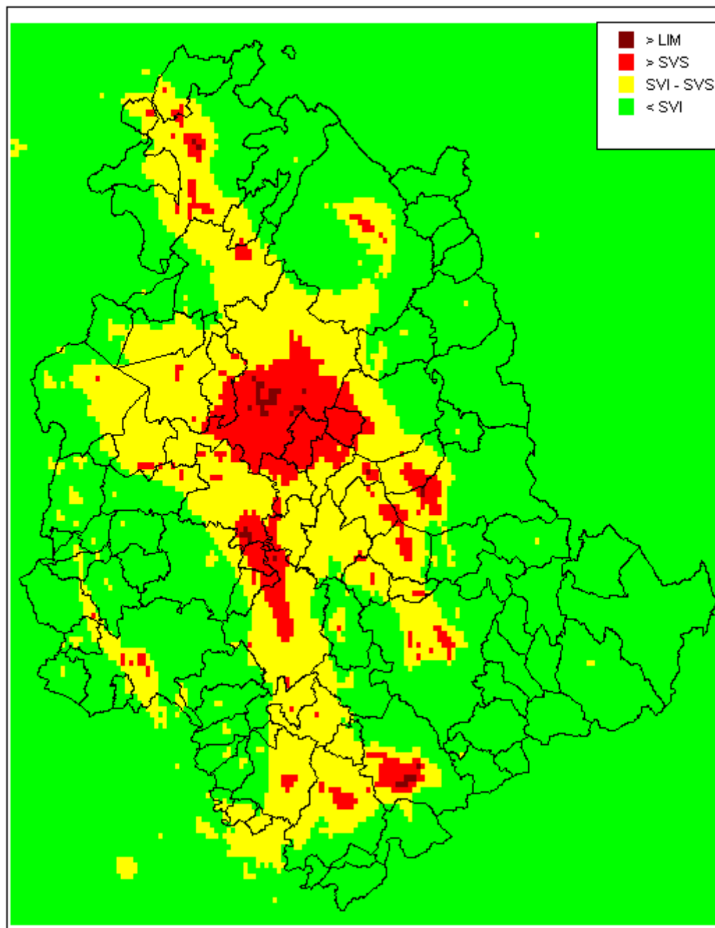
Figura 71 – Stima dei superamenti di soglie di valutazione e valore limite per la media giornaliera del PM 10 valutati con il modello Chimere per l'anno 2025 in Scenario Tendenziale
