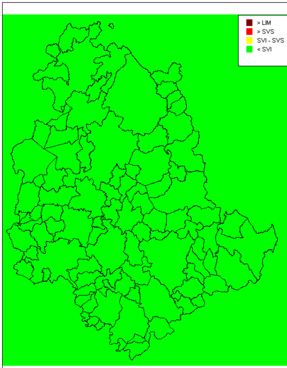
Figura 40 – Stima dei superamenti di soglie di valutazione e valore limite per la media giornaliera degli ossidi di zolfo valutati con il modello Chimere per l'anno 2015
