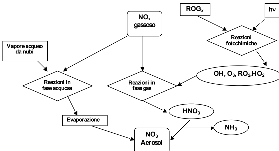
Figura 7 - Trasformazione di NO x in aerosol
