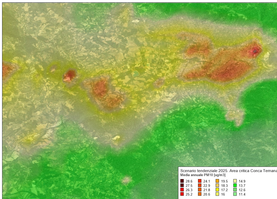
Figura 93 – Media annuale delle concentrazioni di \text{PM}_{10} totale valutate con il modello Chimere ( \mu\text{g}/\text{m}^3 ) per l'anno 2025 in Scenario Tendenziale per l'area critica conca ternana
