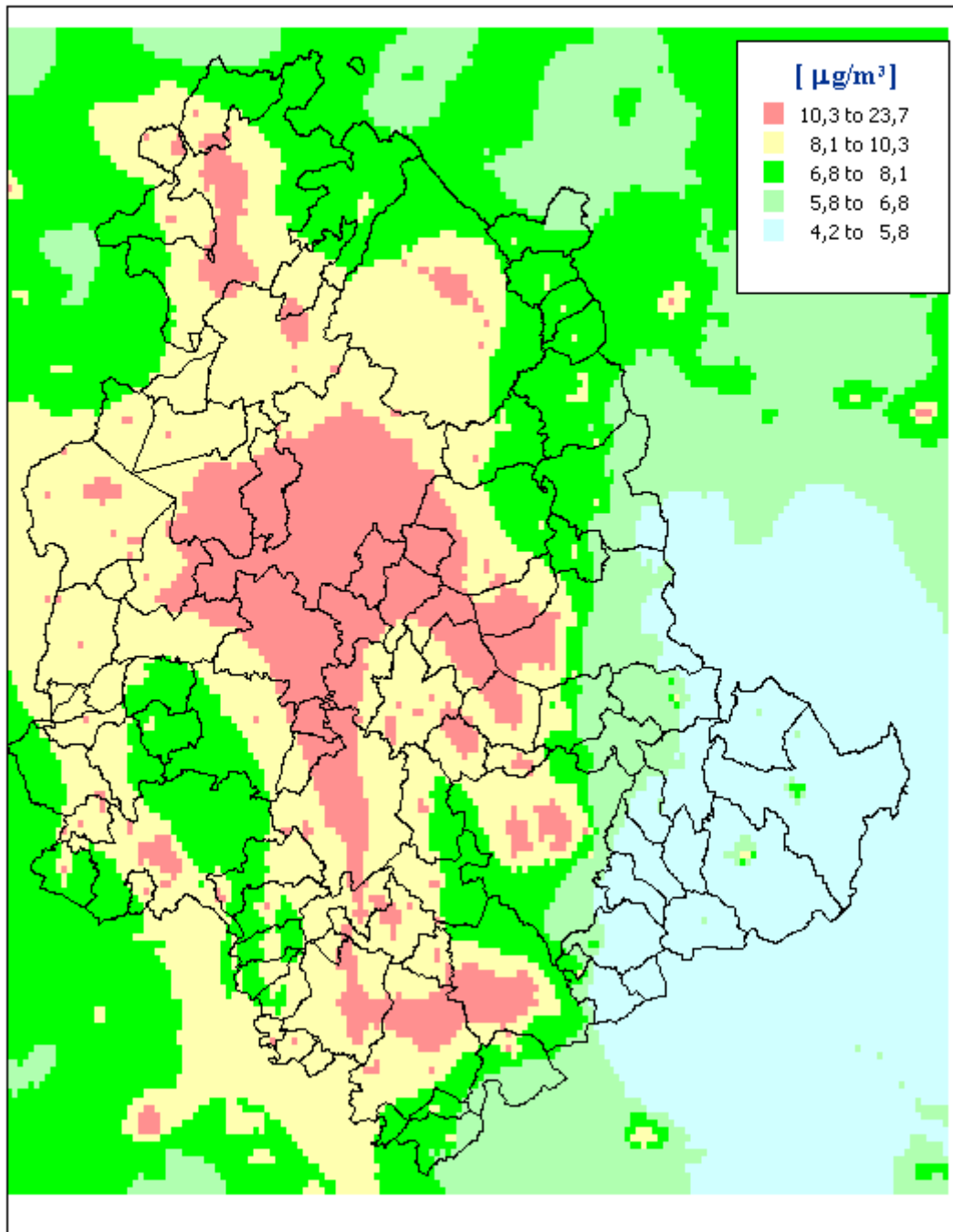
Figura 64 – Media annuale delle concentrazioni di PM 10 antropico valutate con il modello Chimere ( \mu\text{g}/\text{m}^3 ) per l'anno 2025 in Scenario Tendenziale
