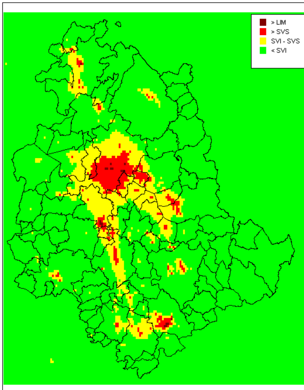
Figura 38 – Stima dei superamenti di soglie di valutazione e valore limite per la media giornaliera del PM 10 antropico valutati con il modello Chimere per l'anno 2015
