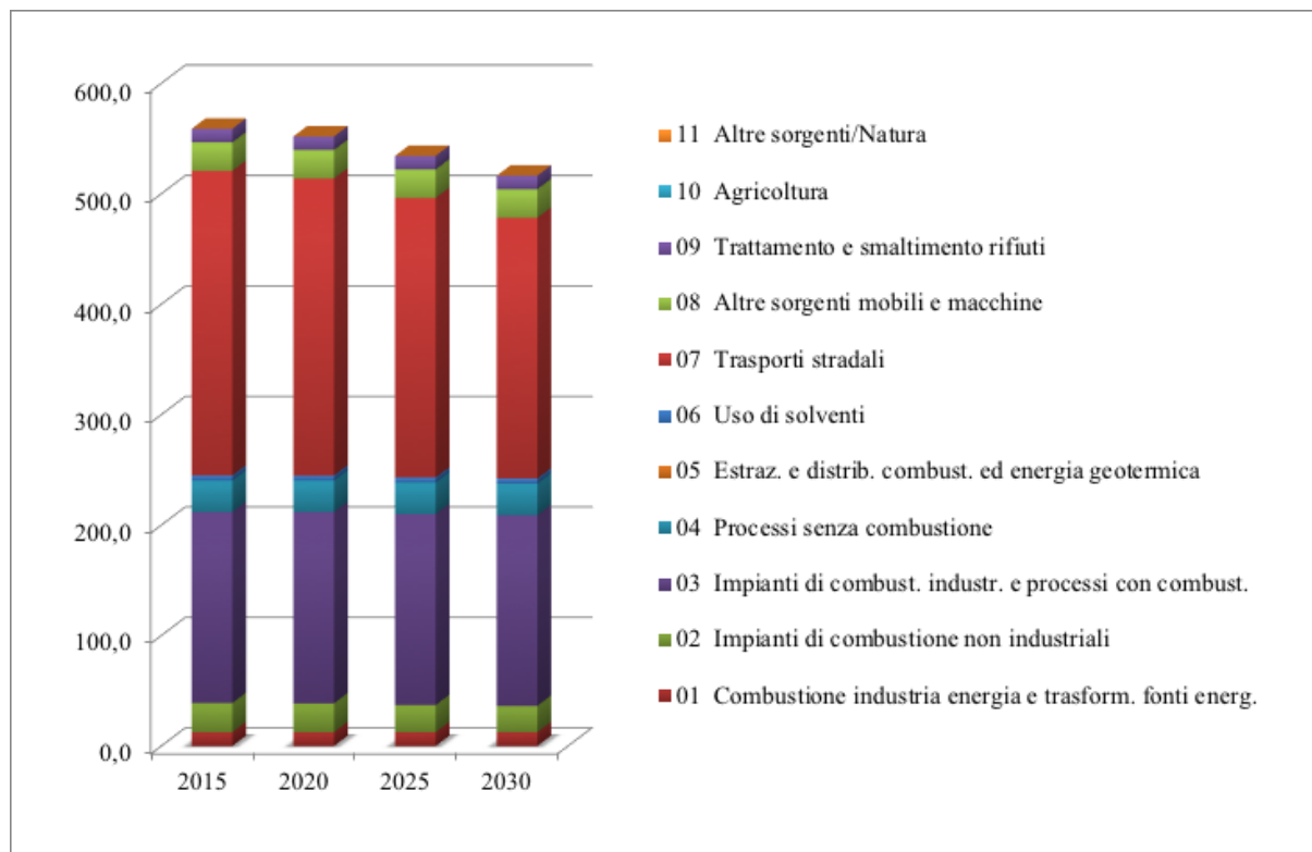
Figura 52 – Andamento delle emissioni totali (Mg) di ossidi di azoto (NO x ) nello scenario tendenziale regionale per il comune di Narni
