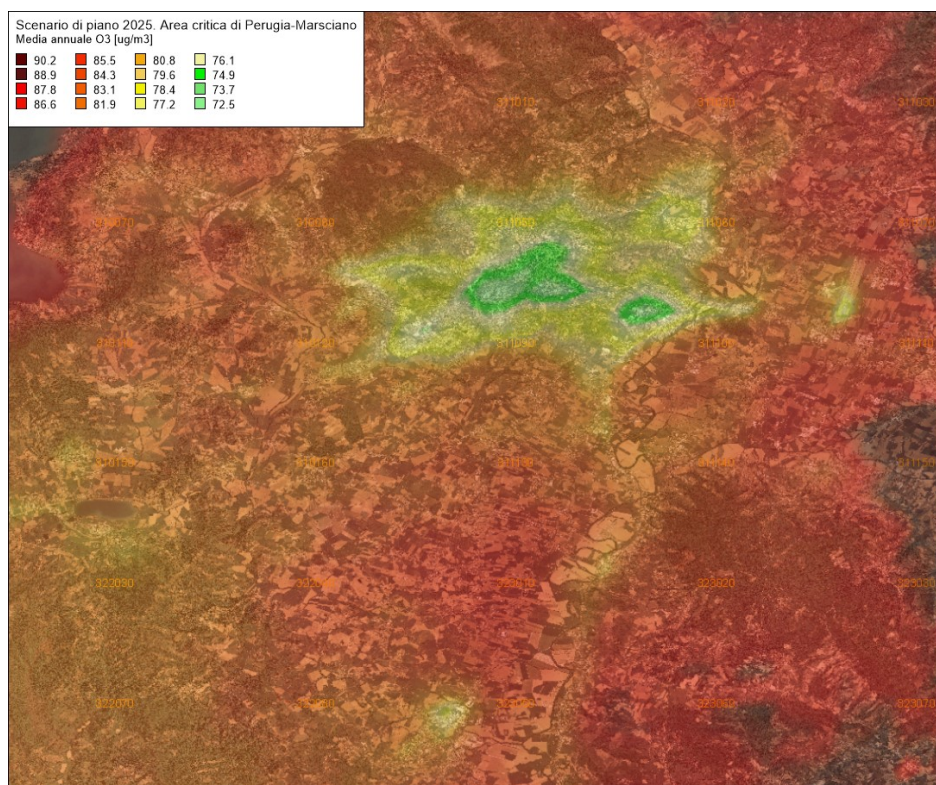
Figura 117 – Media annuale delle concentrazioni di ozono (O 3 ) valutate con il modello Chimere (µg/m³) per l'anno 2025 in Scenario di Piano per l'area critica Perugia e Marsciano
