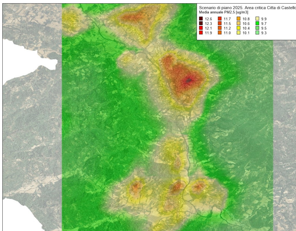
Figura 139 – Media annuale delle concentrazioni di PM 2.5 valutate con il modello Chimere (µg/m 3 ) per l'anno 2025 in Scenario di Piano per l'area critica Città di Castello
