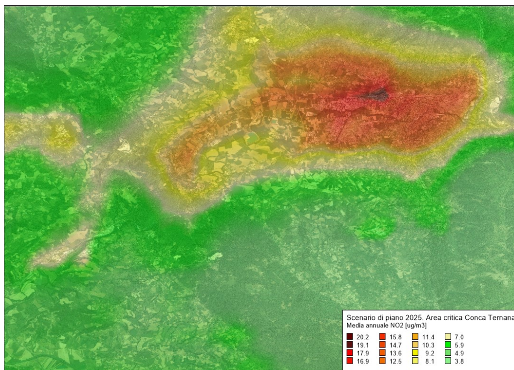
Figura 100 – Media annuale delle concentrazioni di biossido di azoto ( \text{NO}_2 ) valutate con il modello Chimere ( \mu\text{g}/\text{m}^3 ) per l'anno 2025 in Scenario di Piano per l'area critica conca ternana
