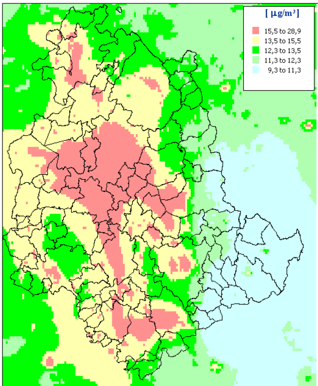
Figura 62 – Media annuale delle concentrazioni di PM 10 totale valutate con il modello Chimere ( \mu\text{g}/\text{m}^3 ) per l'anno 2025 in Scenario Tendenziale
