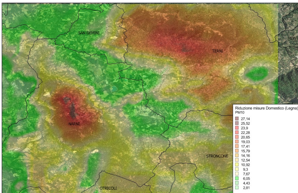
Figura 78 – Stima della riduzione percentuale nella media delle concentrazioni di \text{PM}_{10} valutate con il modello Chimere ( \mu\text{g}/\text{m}^3 ) per l'anno 2020 (Gennaio-Marzo) in Scenario Conca Ternana rispetto all'analogo periodo del 2015: misure sulla combustione legna nel domestico e sulla combustione dei residui agricoli
