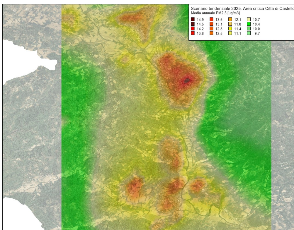
Figura 140 – Media annuale delle concentrazioni di PM 2.5 valutate con il modello Chimere (µg/m 3 ) per l'anno 2025 in Scenario Tendenziale per l'area critica Città di Castello
