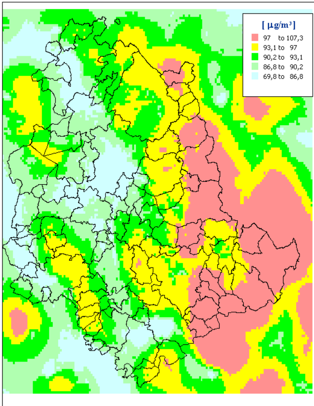
Figura 68 – Media annuale delle concentrazioni di ozono valutate con il modello Chimere ( \mu\text{g}/\text{m}^3 ) per l'anno 2025 in Scenario Tendenziale
