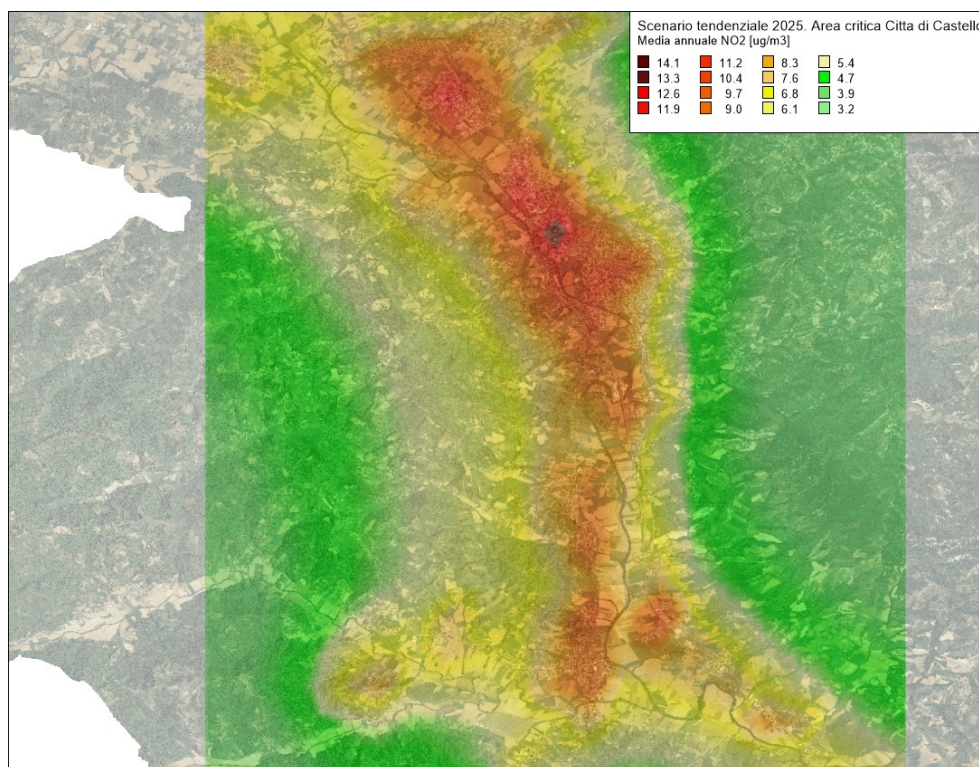
Figura 143 – Media annuale delle concentrazioni di biossido di azoto (NO 2 ) valutate con il modello Chimere (µg/m 3 ) per l'anno 2025 in Scenario Tendenziale per l'area critica Città di Castello
