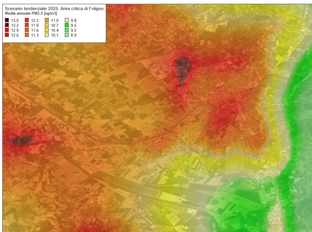
Figura 126 – Media annuale delle concentrazioni di PM 2,5 valutate con il modello Chimere (µg/m 3 ) per l'anno 2025 in Scenario Tendenziale per l'area critica Foligno
