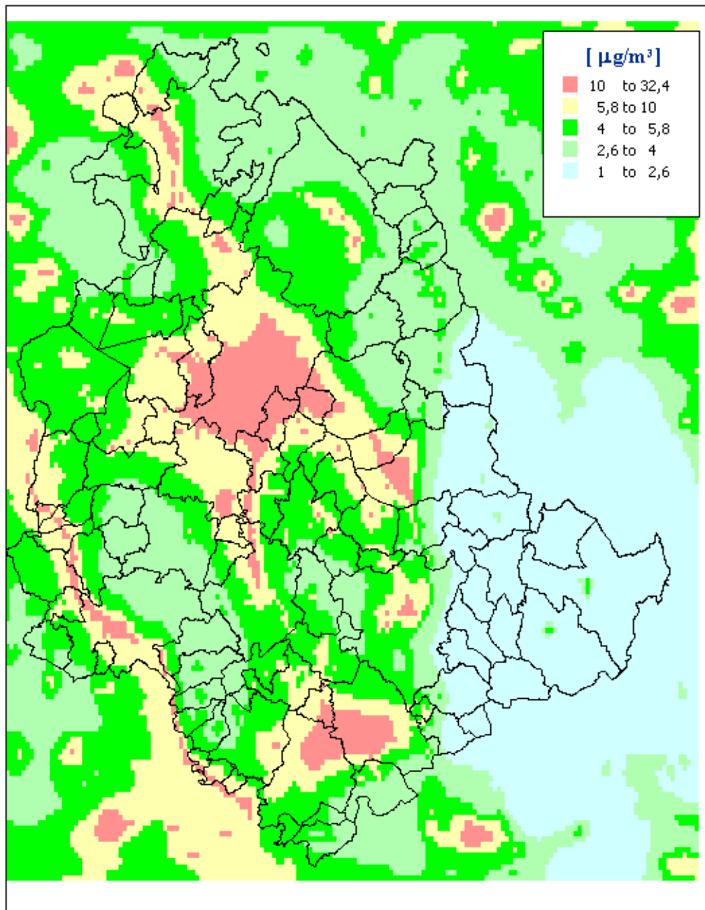
Figura 26 – Media annuale delle concentrazioni di biossido di azoto (NO 2 ) valutate con il modello Chimere (µg/m 3 ) per l'anno 2015
