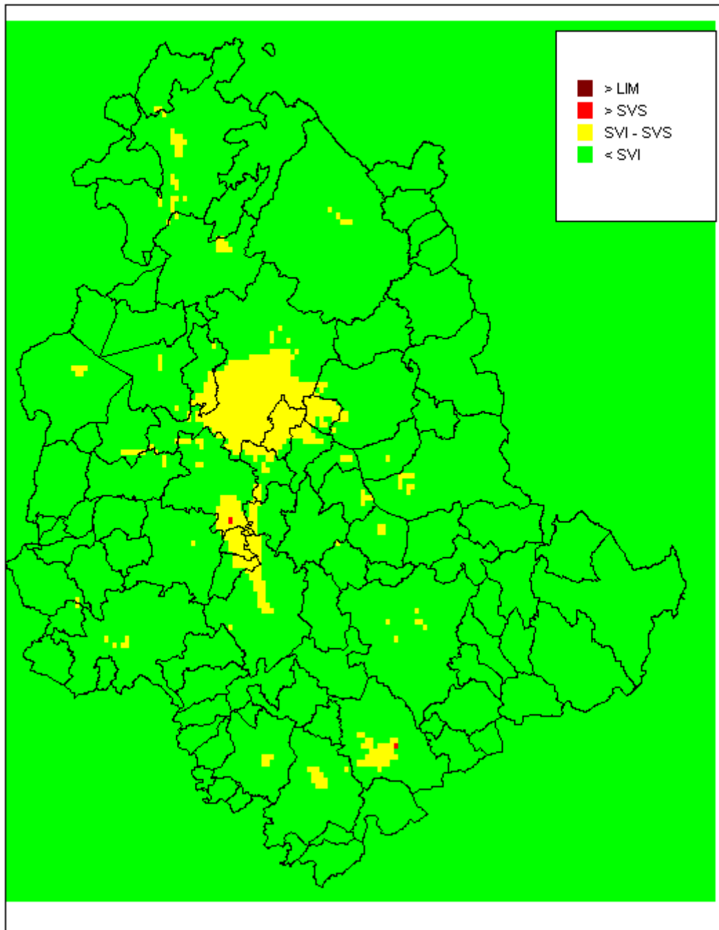
Figura 67 – Media annuale delle concentrazioni di PM 2,5 valutate con il modello Chimere per l'anno 2025 in Scenario Tendenziale con riferimento alle soglie legislative
