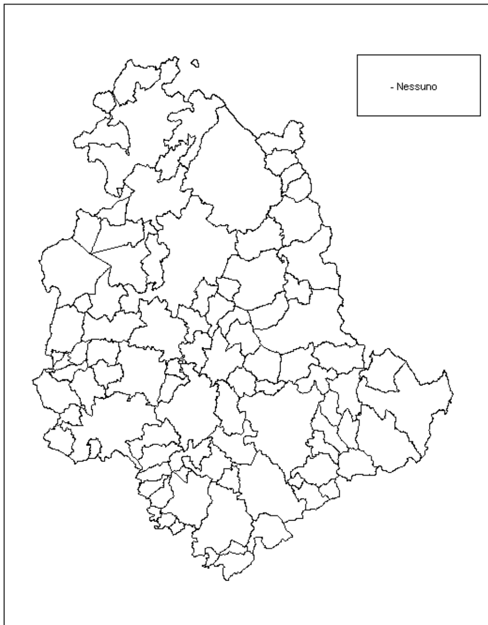
Figura 41 – Stima dei superamenti del valore limite per la media oraria degli ossidi di zolfo valutati con il modello Chimere per l'anno 2015
