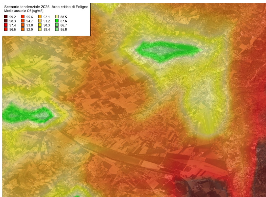
Figura 132 – Media annuale delle concentrazioni di ozono (O 3 ) valutate con il modello Chimere (µg/m 3 ) per l'anno 2025 in Scenario Tendenziale per l'area critica Foligno
