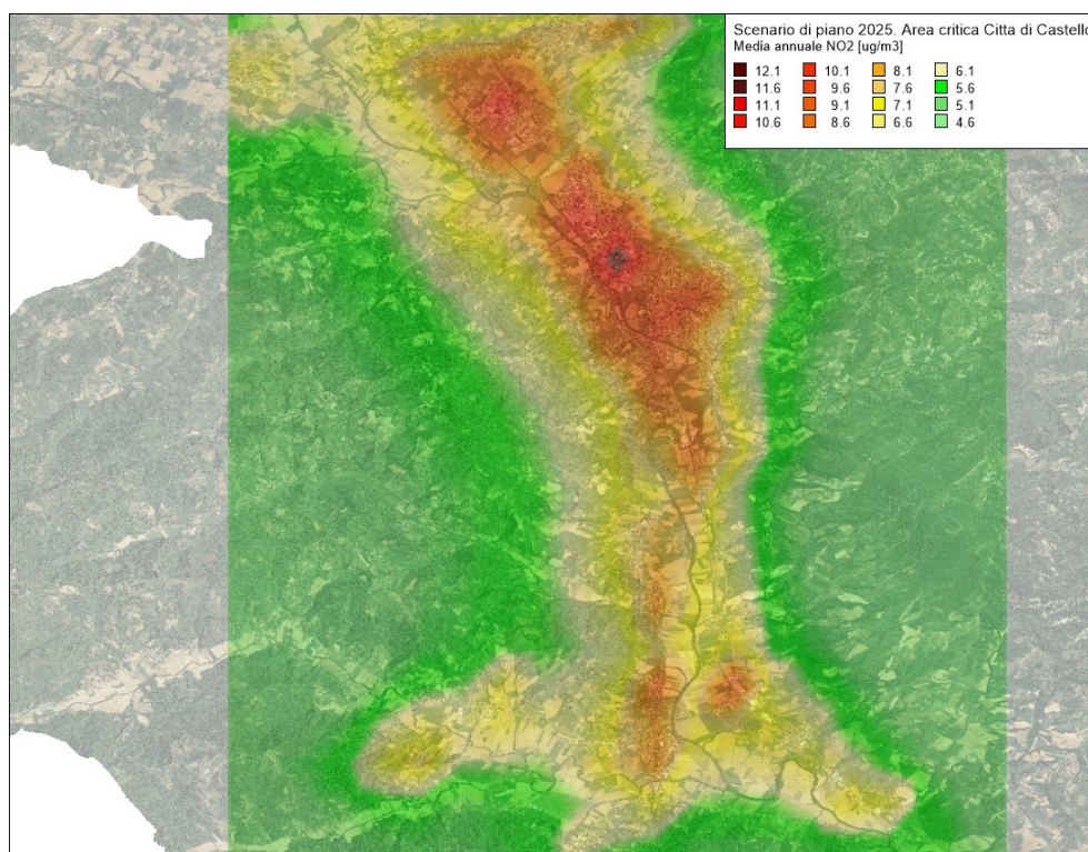
Figura 142 – Media annuale delle concentrazioni di biossido di azoto (NO 2 ) valutate con il modello Chimere (µg/m 3 ) per l'anno 2025 in Scenario di Piano per l'area critica Città di Castello
