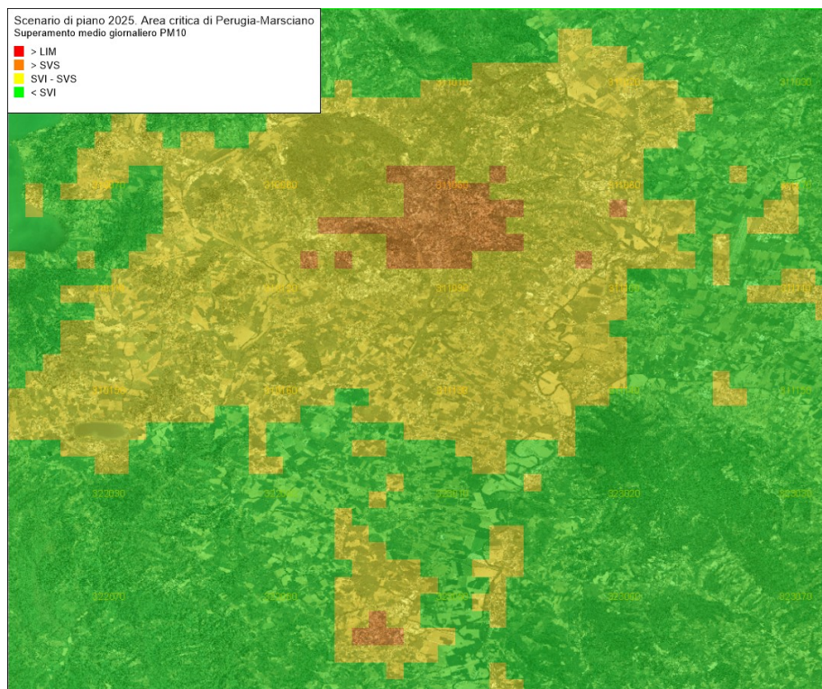
Figura 109 – Superamenti della media giornaliera delle concentrazioni di PM 10 valutate con il modello Chimere ( \mu\text{g}/\text{m}^3 ) per l'anno 2025 in Scenario di Piano per l'area critica Perugia e Marsciano
