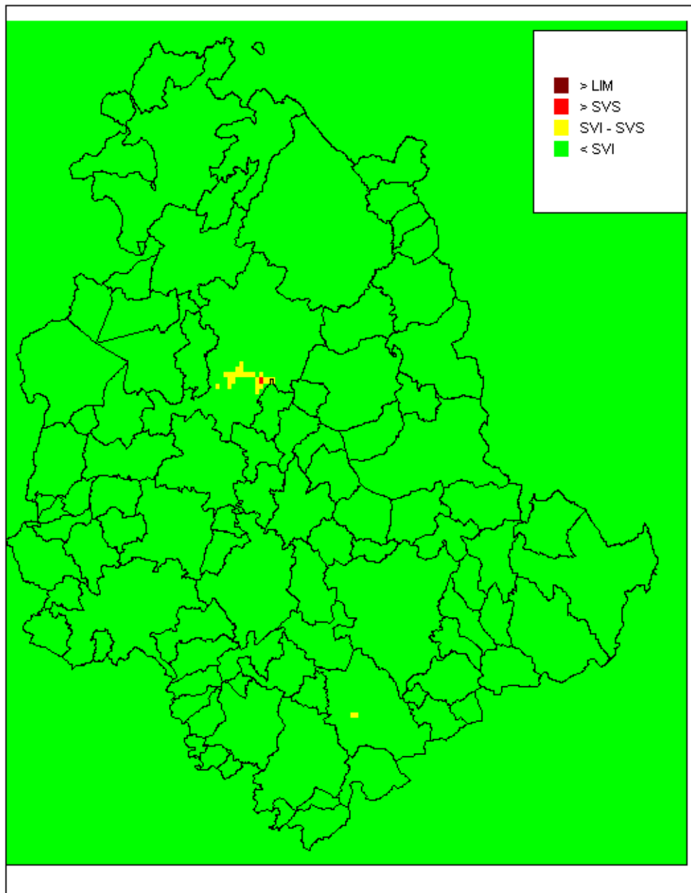
Figura 27 – Media annuale delle concentrazioni di biossido di azoto (NO 2 ) valutate con il modello Chimere per l'anno 2015 con riferimento alle soglie legislative
