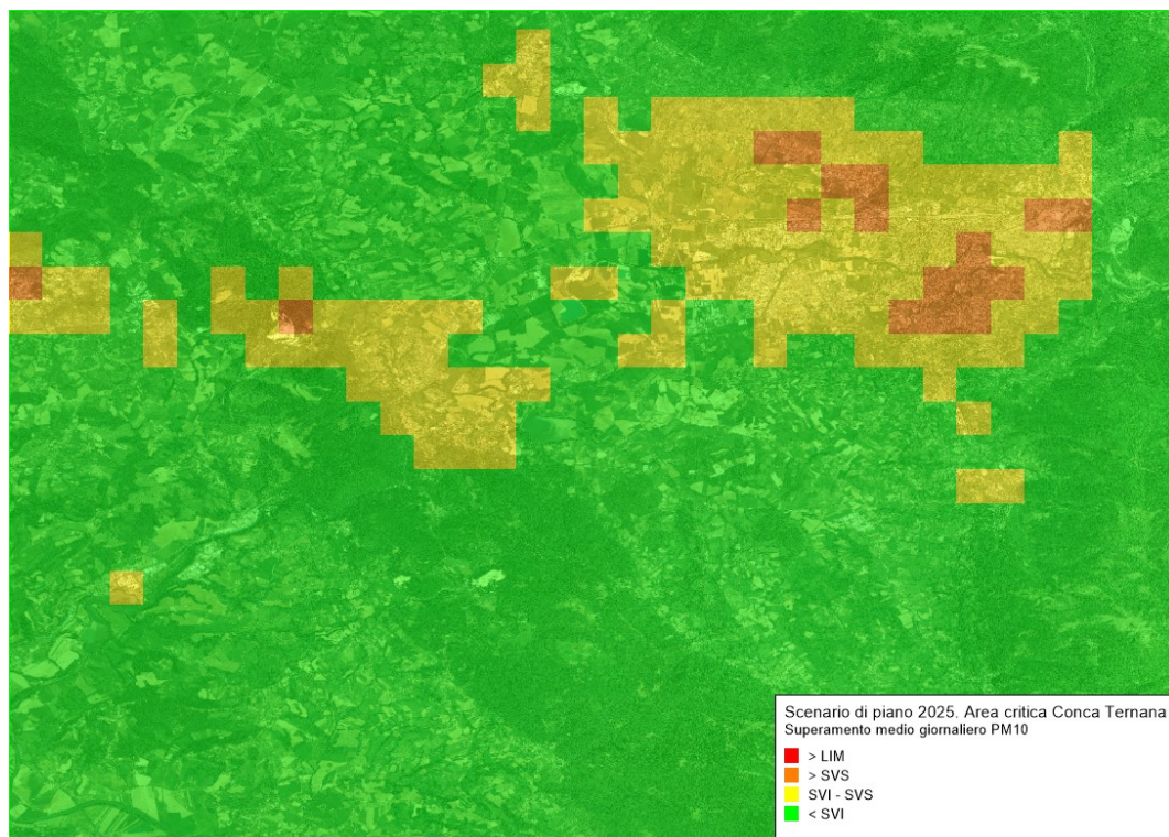
Figura 95 – Superamenti della media giornaliera delle concentrazioni di PM 10 valutate con il modello Chimere ( \mu\text{g}/\text{m}^3 ) per l'anno 2025 in Scenario di Piano per l'area critica conca ternana
