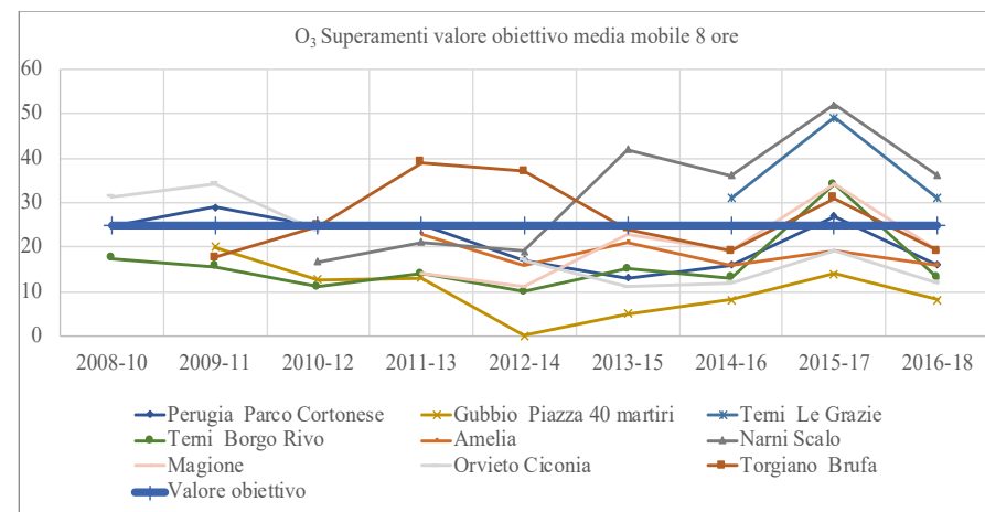
Figura 16 - Rete di rilevamento della qualità dell'aria: Superamenti media mobile 8 ore O 3
