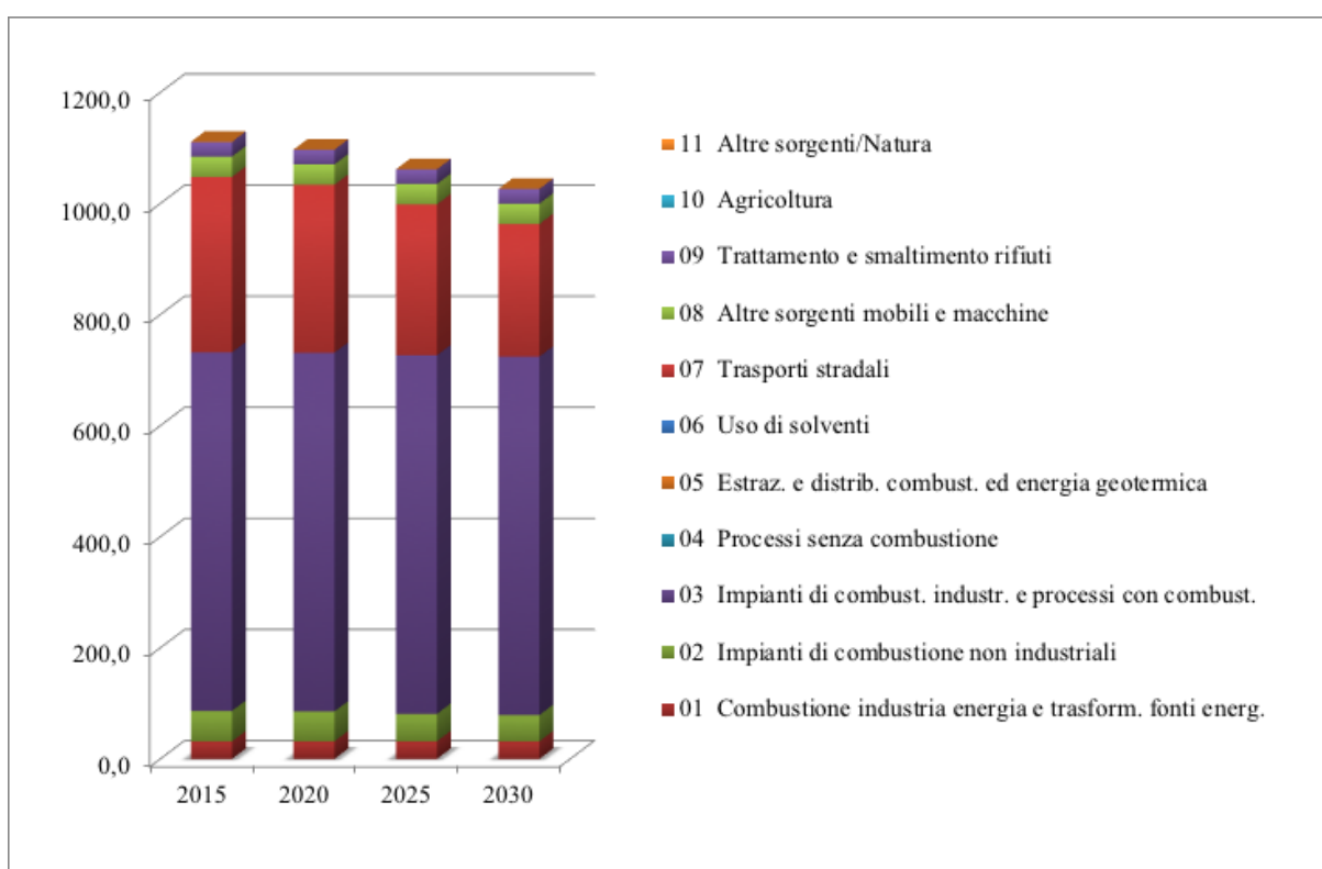
Figura 58 – Andamento delle emissioni totali (Mg) di ossidi di azoto (NO x ) nello scenario tendenziale regionale per il comune di Spoleto
