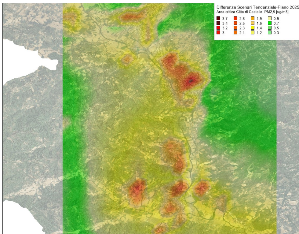
Figura 141 – Riduzione nella media annuale delle concentrazioni di PM 2.5 valutate con il modello Chimere (µg/m 3 ) per l'anno 2025 in Scenario di Piano rispetto allo Scenario Tendenziale per l'area critica Città di Castello
