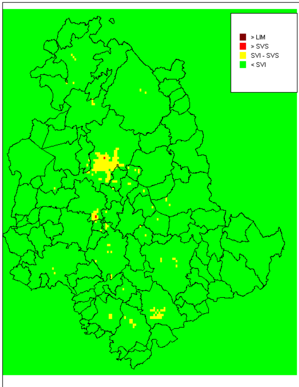
Figura 29 – Media annuale delle concentrazioni di PM 10 totale valutate con il modello Chimere per l'anno 2015 con riferimento alle soglie legislative
