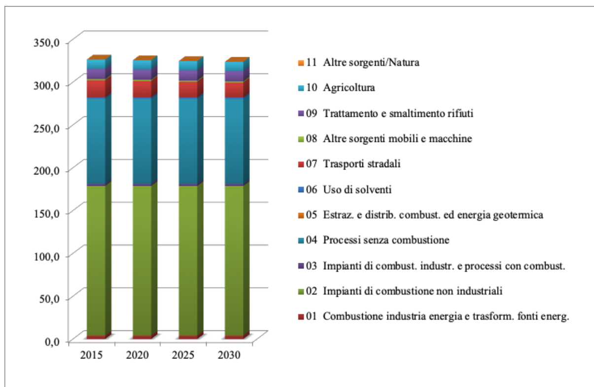
Figura 53 – Andamento delle emissioni totali (Mg) di particelle con diametro inferiore a 10 micron (PM 10 ) nello scenario tendenziale regionale per il comune di Narni
