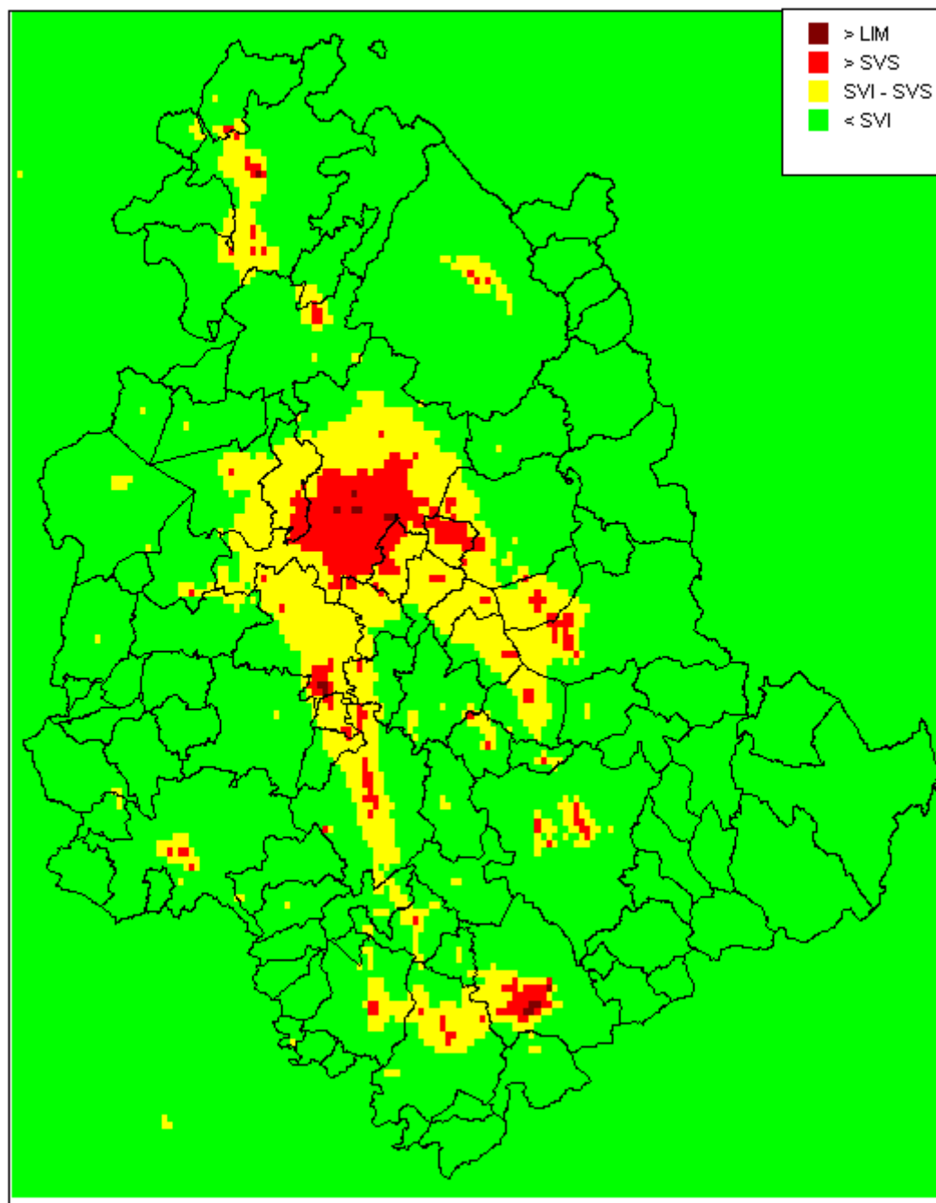
Figura 72 – Stima dei superamenti di soglie di valutazione e valore limite per la media giornaliera del PM 10 antropico valutati con il modello Chimere per l'anno 2025 in Scenario Tendenziale
