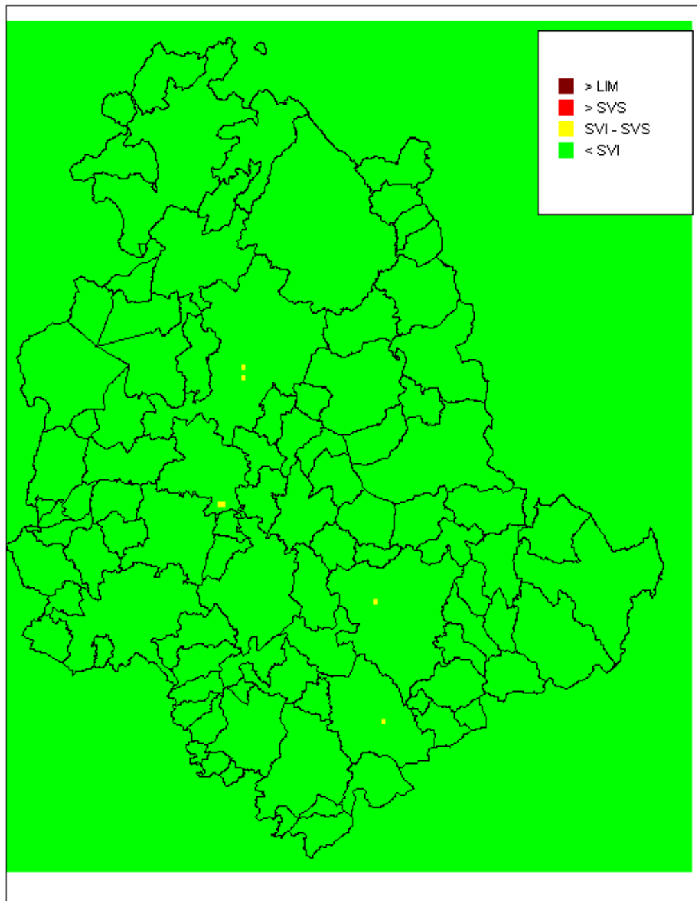
Figura 31 – Media annuale delle concentrazioni di PM 10 antropico valutate con il modello Chimere per l'anno 2015 con riferimento alle soglie legislative
