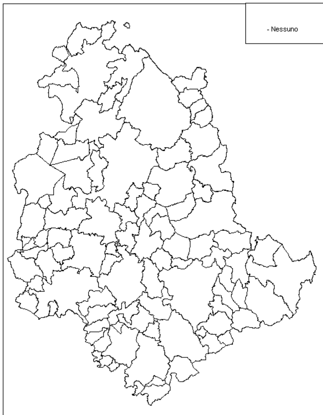
Figura 75 – Stima dei superamenti del valore limite per la media oraria degli ossidi di zolfo valutati con il modello Chimere per l'anno 2025 in Scenario Tendenziale
