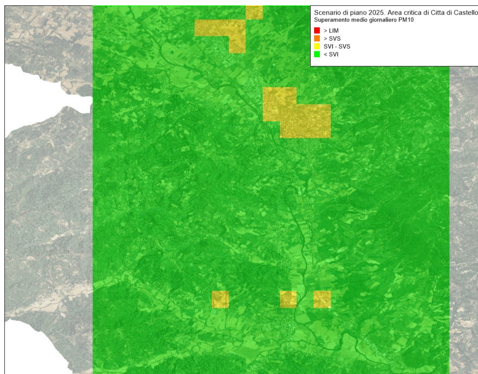
Figura 137 – Superamenti della media giornaliera delle concentrazioni di PM 10 valutate con il modello Chimere ( \mu\text{g}/\text{m}^3 ) per l'anno 2025 in Scenario di Piano per l'area critica Città di Castello
