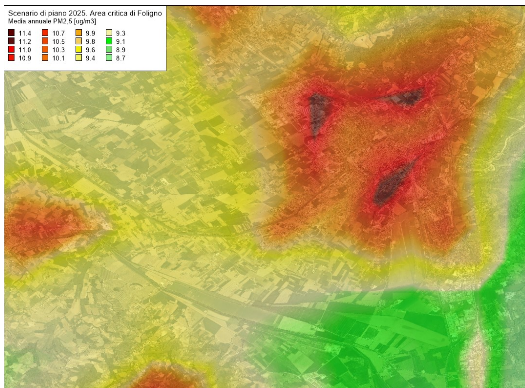
Figura 125 – Media annuale delle concentrazioni di PM 2,5 valutate con il modello Chimere (µg/m 3 ) per l'anno 2025 in Scenario di Piano per l'area critica Foligno
