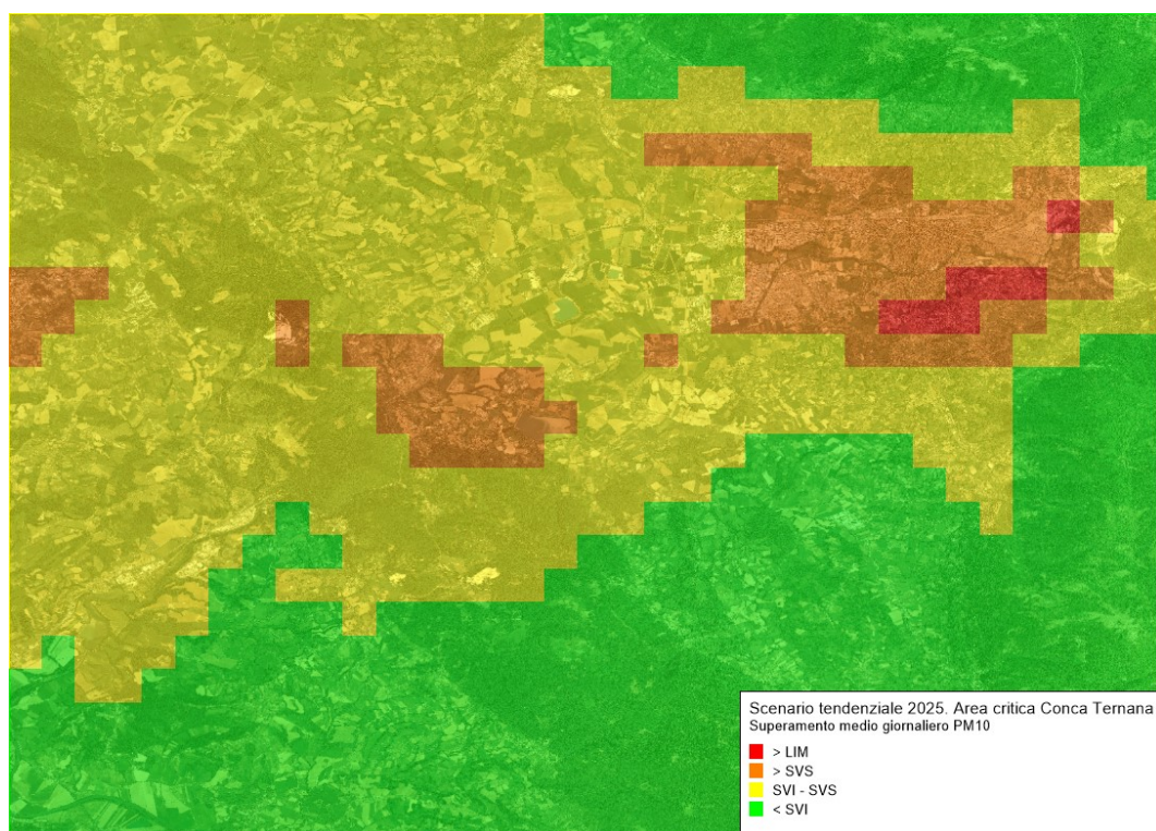
Figura 96 – Superamenti della media giornaliera di PM 10 valutate con il modello Chimere ( \mu\text{g}/\text{m}^3 ) per l'anno 2025 in Scenario Tendenziale per l'area critica conca ternana
