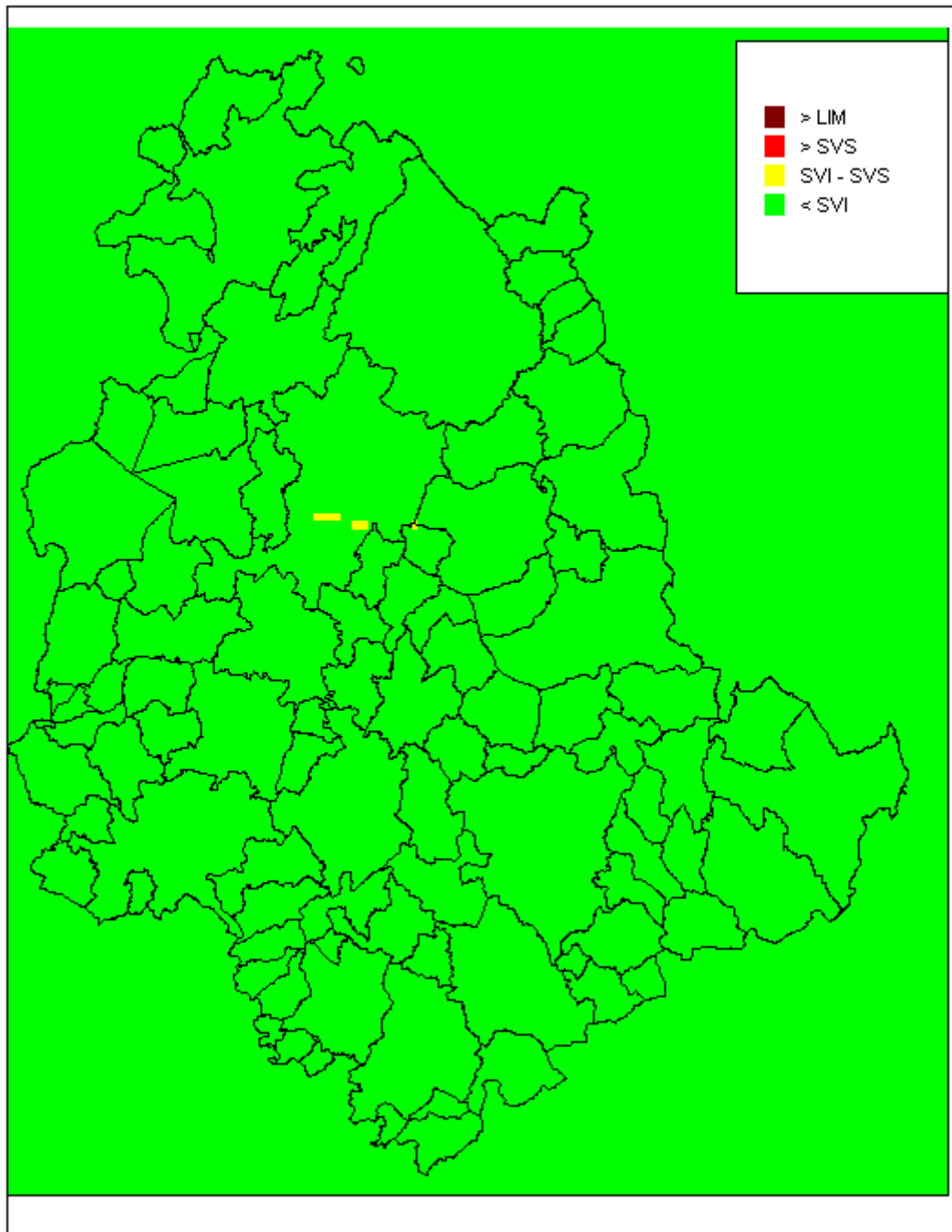
Figura 61 – Media annuale delle concentrazioni di biossido di azoto (NO 2 ) valutate con il modello Chimere per l'anno 2025 in Scenario Tendenziale con riferimento alle soglie legislative
