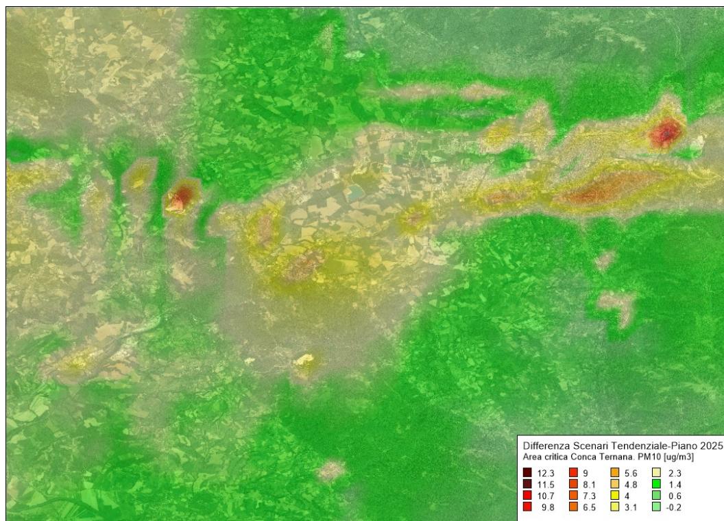
Figura 99 – Riduzione nella media annuale delle concentrazioni di \text{PM}_{2.5} totale valutate con il modello Chimere ( \mu\text{g}/\text{m}^3 ) per l'anno 2025 in Scenario Tendenziale per l'area critica conca ternana
