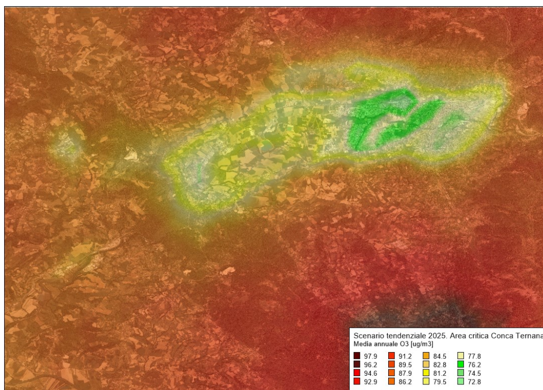
Figura 104 – Media annuale delle concentrazioni di ozono (O 3 ) valutate con il modello Chimere (µg/m 3 ) per l'anno 2025 in Scenario Tendenziale per l'area critica conca ternana
