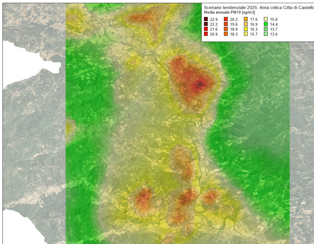
Figura 135 – Media annuale delle concentrazioni di PM 10 totale valutate con il modello Chimere ( \mu\text{g}/\text{m}^3 ) per l'anno 2025 in Scenario Tendenziale per l'area critica Città di Castello
