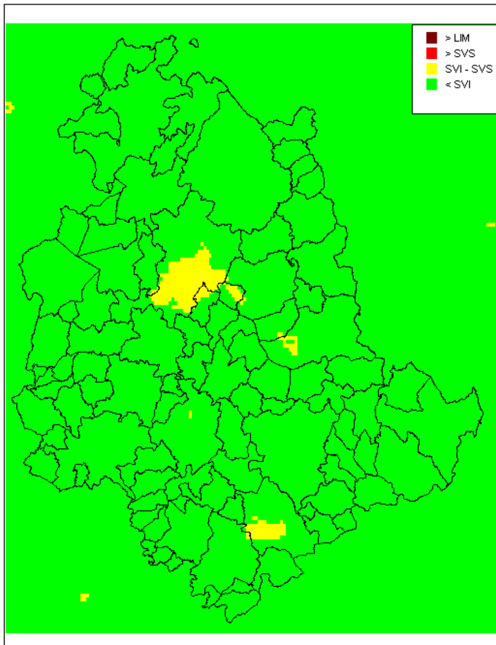
Figura 36 – Stima dei superamenti di soglie di valutazione e valore limite stabilite per la media oraria del biossido di azoto valutati con il modello Chimere per l'anno 2015
