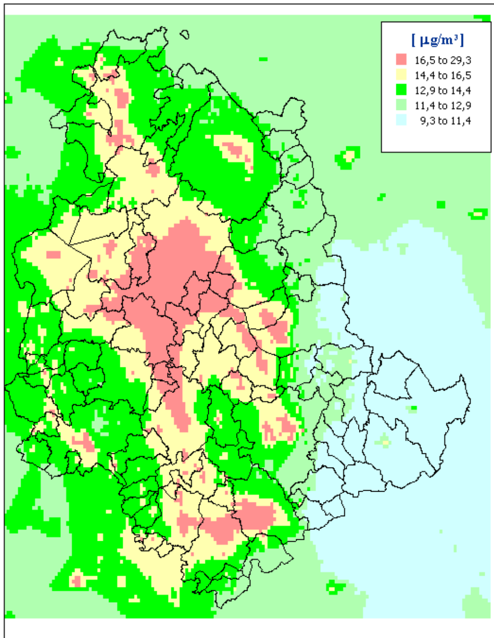
Figura 28 – Media annuale delle concentrazioni di PM 10 totale valutate con il modello Chimere (µg/m³) per l'anno 2015
