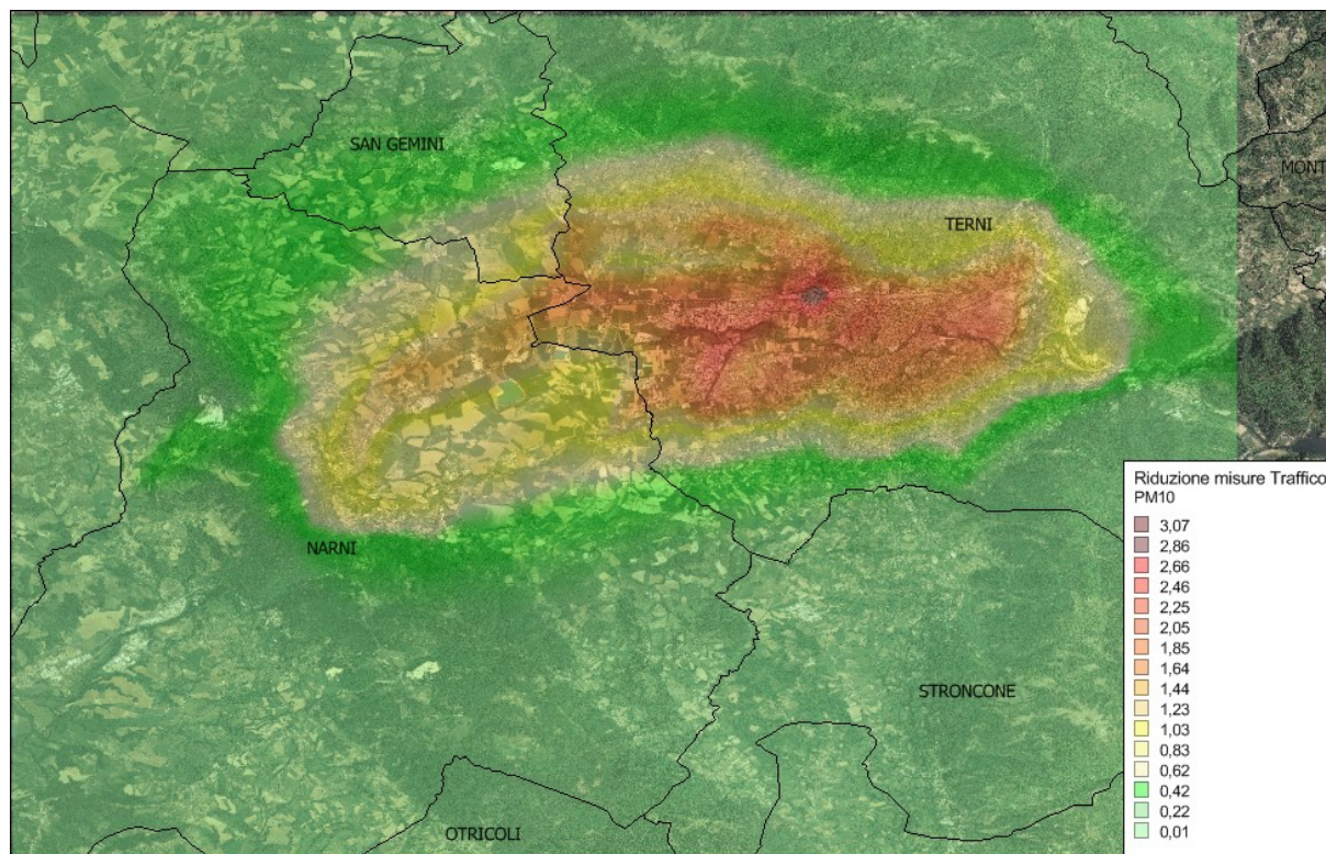
Figura 79 – Stima della riduzione percentuale nella media delle concentrazioni di PM 10 valutate con il modello Chimere ( \mu\text{g}/\text{m}^3 ) per l'anno 2020 (Gennaio-Marzo) in Scenario Conca Ternana rispetto all'analogo periodo del 2015: misure sul traffico
