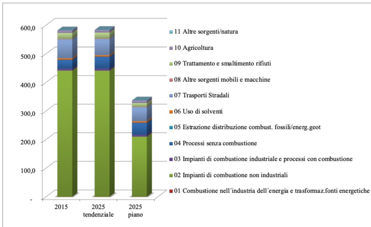
Figura 84 – Andamento delle emissioni totali (Mg) di particelle con diametro inferiore a 10 micron (PM 10 ) negli scenari tendenziale regionale e di piano per il comune di Terni
