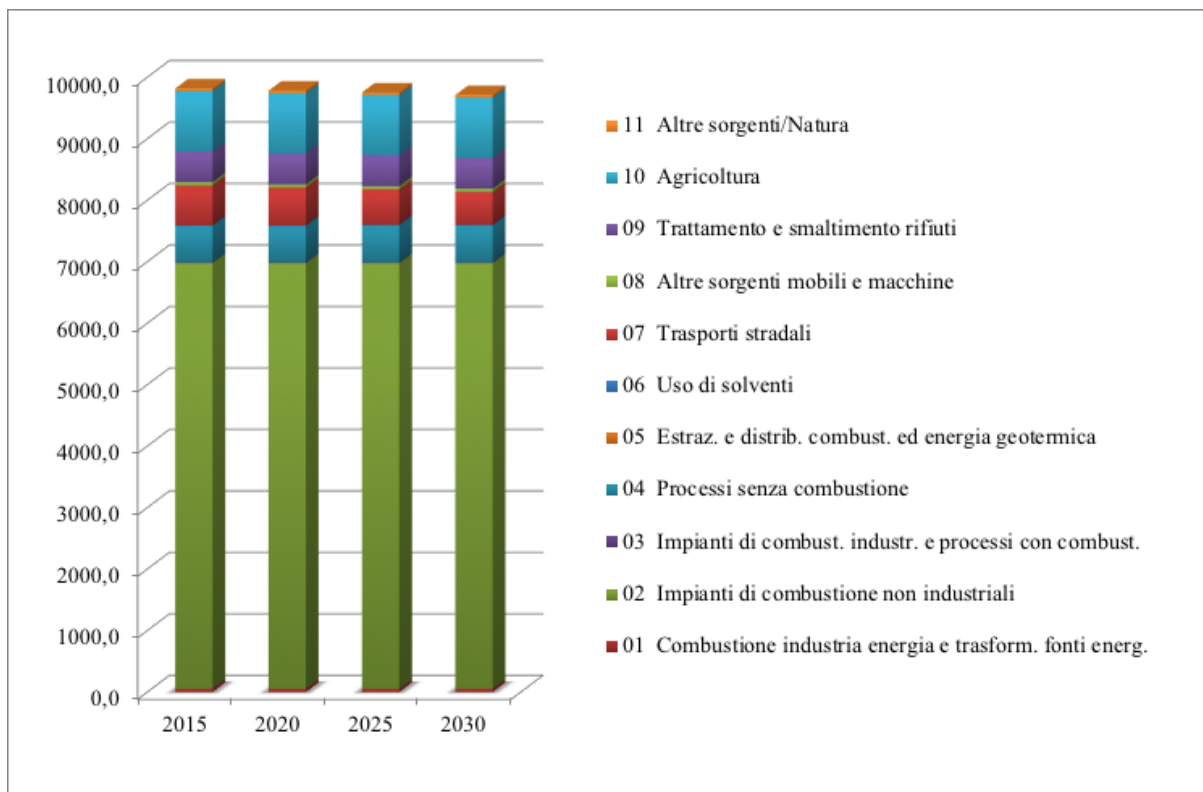
Figura 43 – Andamento delle emissioni totali (Mg) di particelle con diametro inferiore a 10 micron (PM 10 ) nello scenario tendenziale regionale
