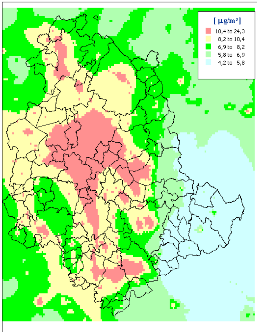
Figura 30 – Media annuale delle concentrazioni di PM 10 antropico valutate con il modello Chimere (µg/m 3 ) per l'anno 2015
