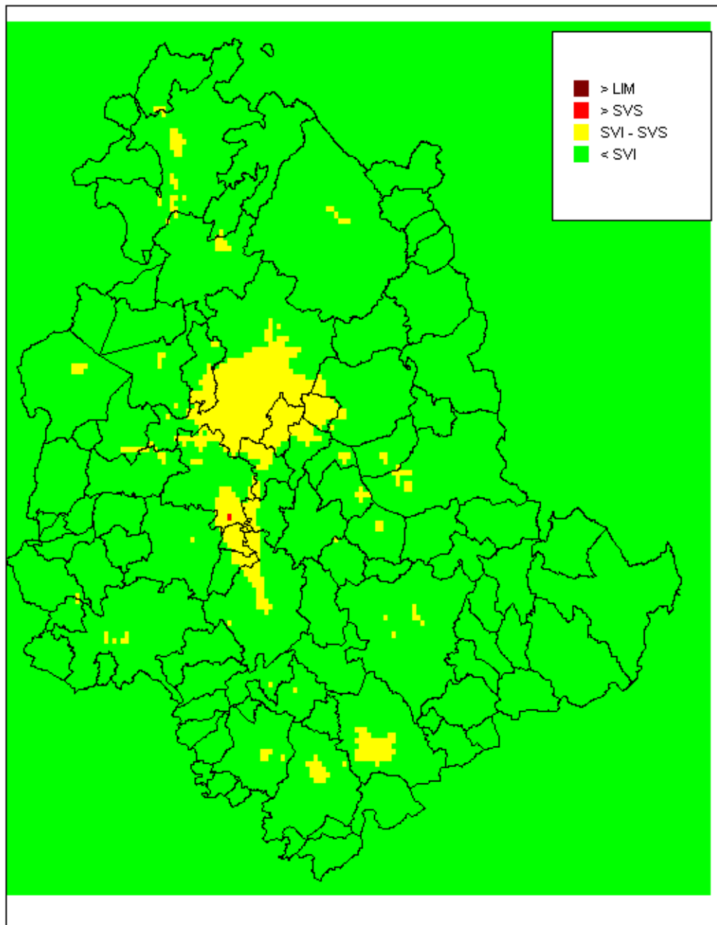
Figura 33 – Media annuale delle concentrazioni di PM 2,5 valutate con il modello Chimere per l'anno 2015 con riferimento alle soglie legislative
